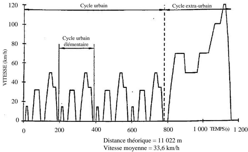
Figure 1 Cycle d'essai du NEDC
