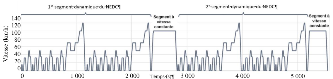
Figure 3a Séquence d'essai abrégée du NEDC
