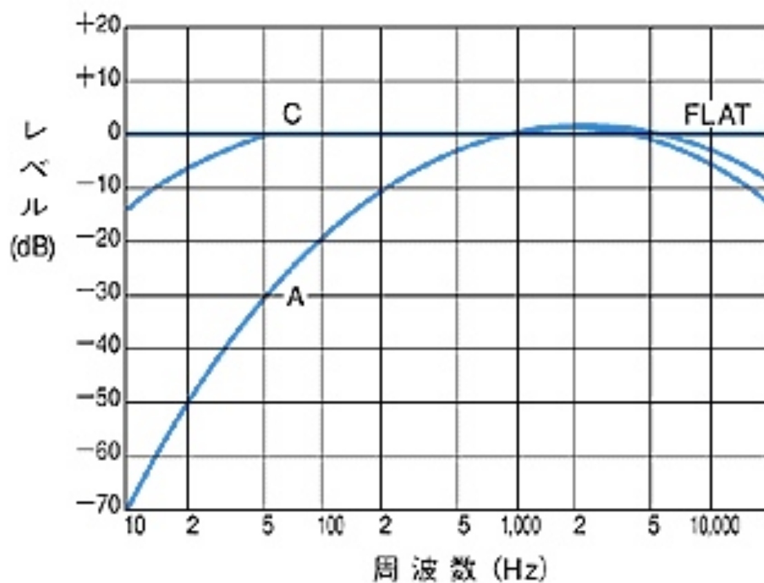
騒音計の周波数重み付け特性
