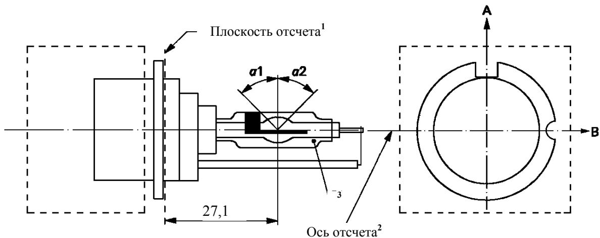
Рис. 3 - Категория D3R - Типовой газоразрядный источник света с пусковым устройством - Цоколь PK32d-6
