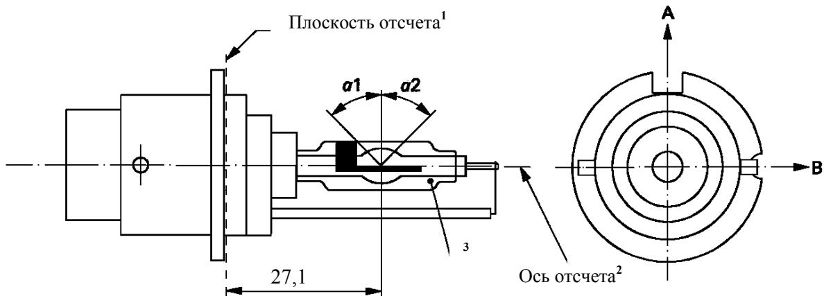
Рис. 4 - Категория D4R - Типовой газоразрядный источник света с соединительным устройством - Цоколь P32d-6
