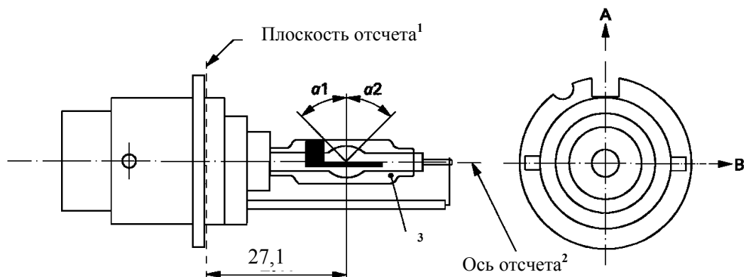
Рис. 2 - Категория D2R - Типовой газоразрядный источник света с соединительным устройством - Цоколь P32d-3
