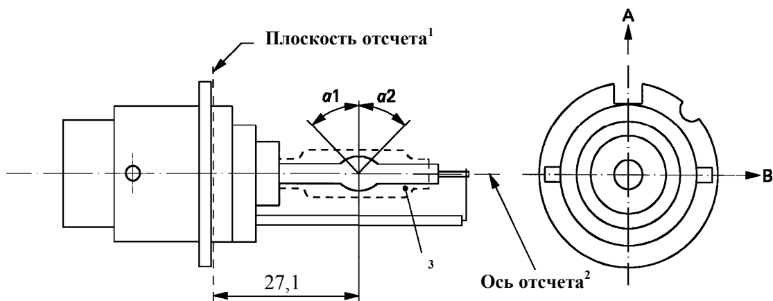
Рис. 2 - Категория D2S - Типовой газоразрядный источник света с соединительным устройством - Цоколь P32d-2
