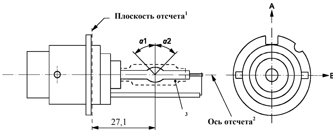
Рис. 4 - Категория D4S - Типовой газоразрядный источник света с соединительным устройством - Цоколь P32d-5
