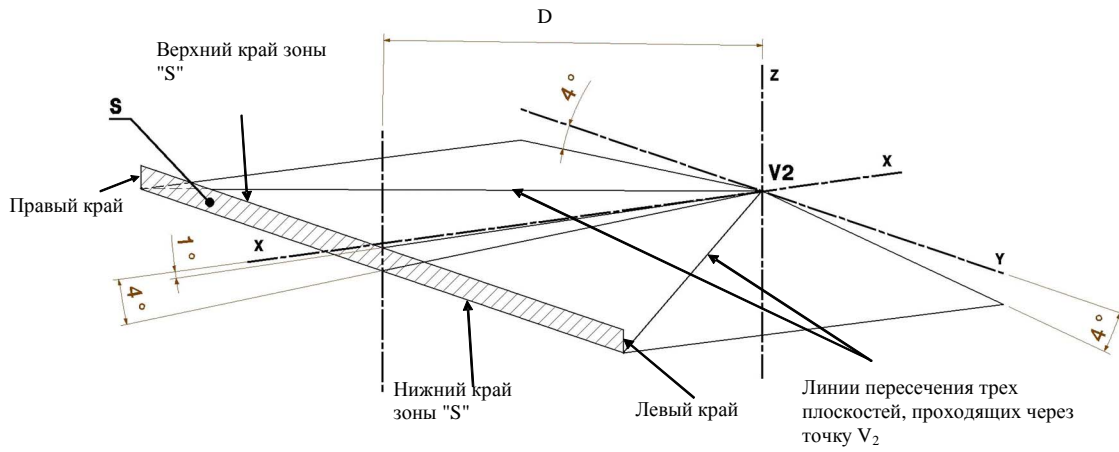
Рис. 7 Определение зоны "S" (пункт 5.1.3.2)
