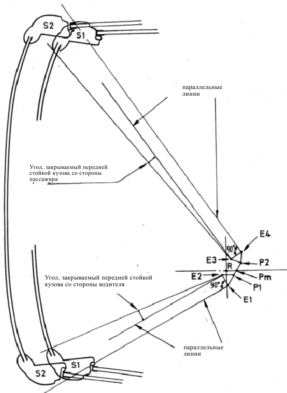
Рис.3 Закрытые углы
