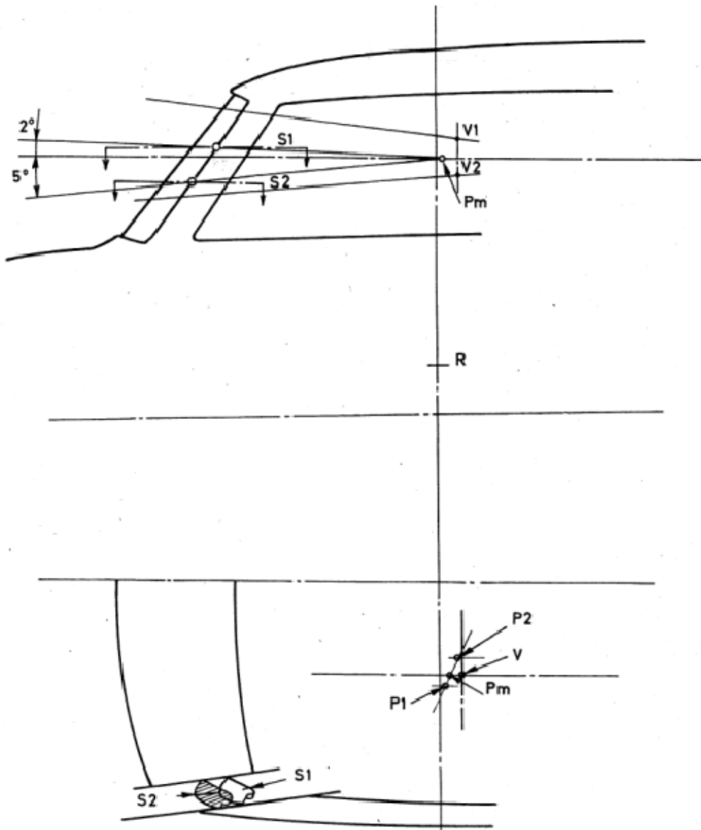
Рис. 2 Точки обзора передних стоек кузова
