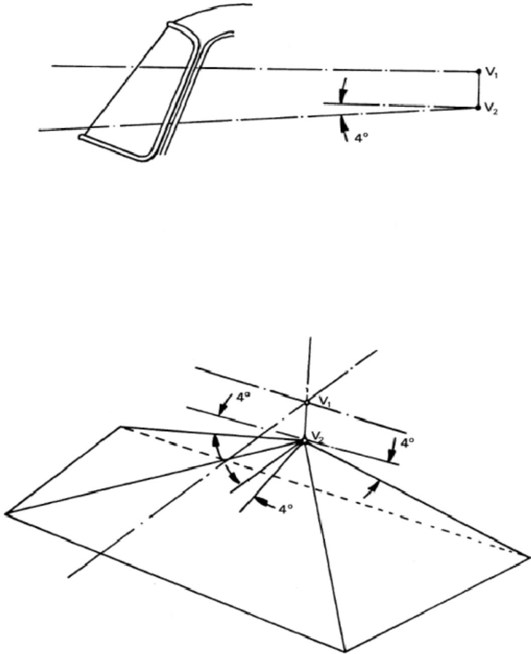
Рис.4 Оценка помех в 180°-ном поле обзора водителя спереди
