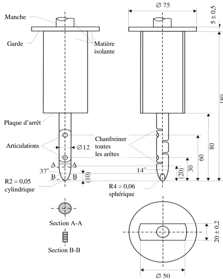
Figure 1 Doigt d'épreuve articulé
