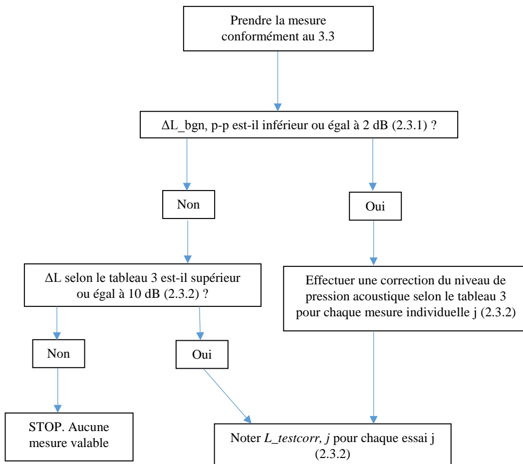
Figure 5 Critères de correction des mesures du niveau de pression acoustique pondéré A du véhicule
