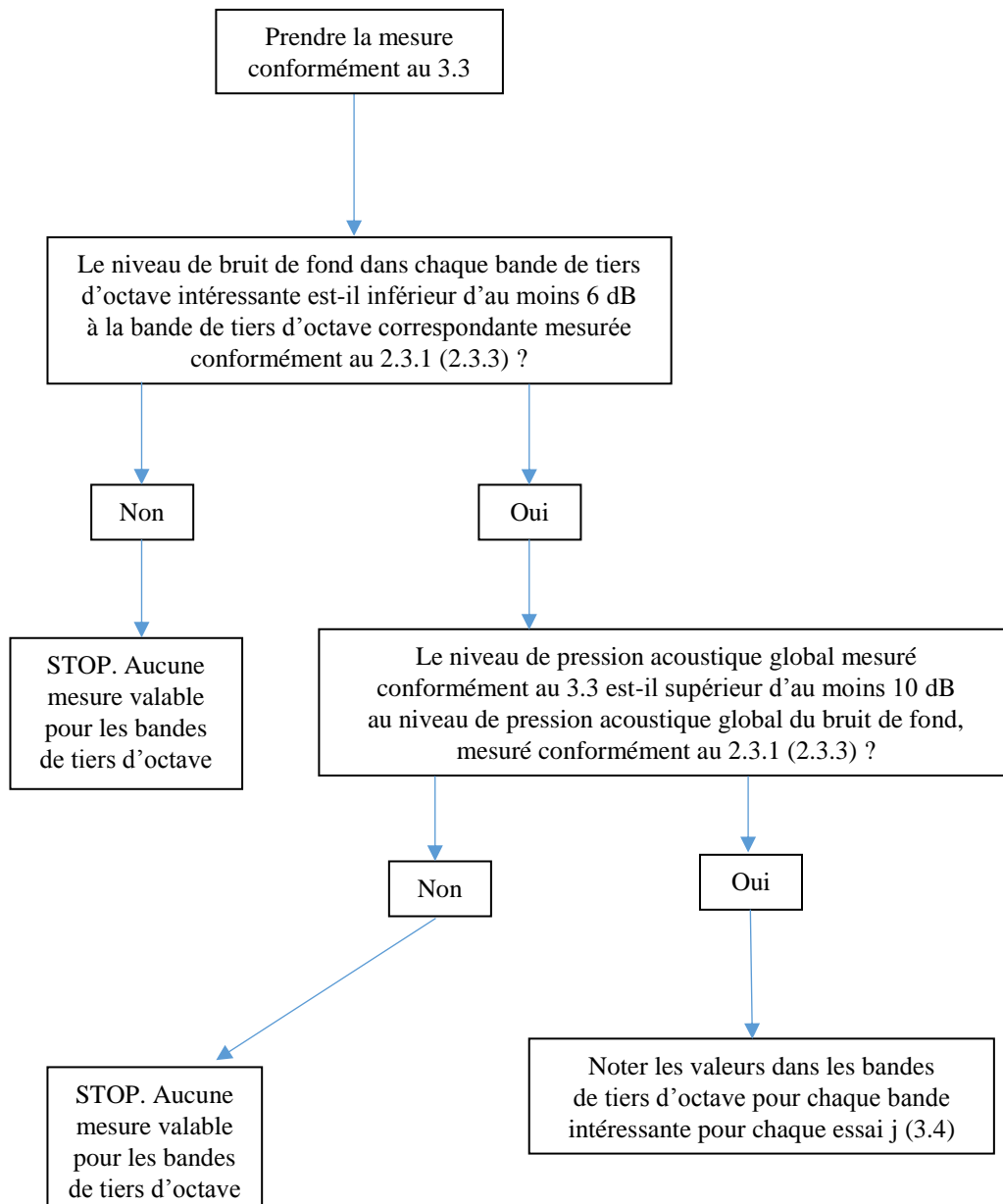
Figure 6 Prescriptions relatives au bruit de fond pour l'analyse dans les bandes de tiers d'octave
