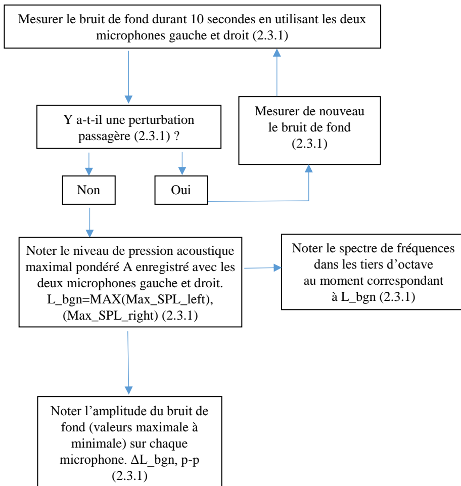
Figure 4 Détermination de l'amplitude du bruit de fond
