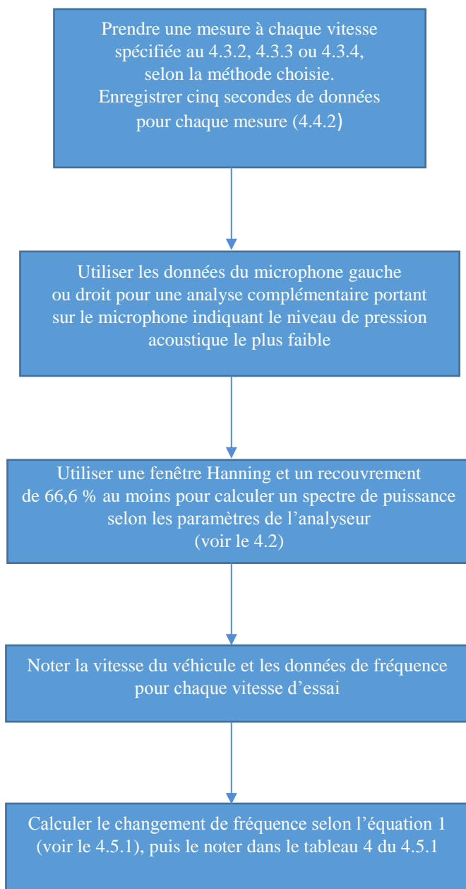
Figure 7c Procédure d'essai pour la mesure du changement de fréquence – méthodes B, C, D et E
