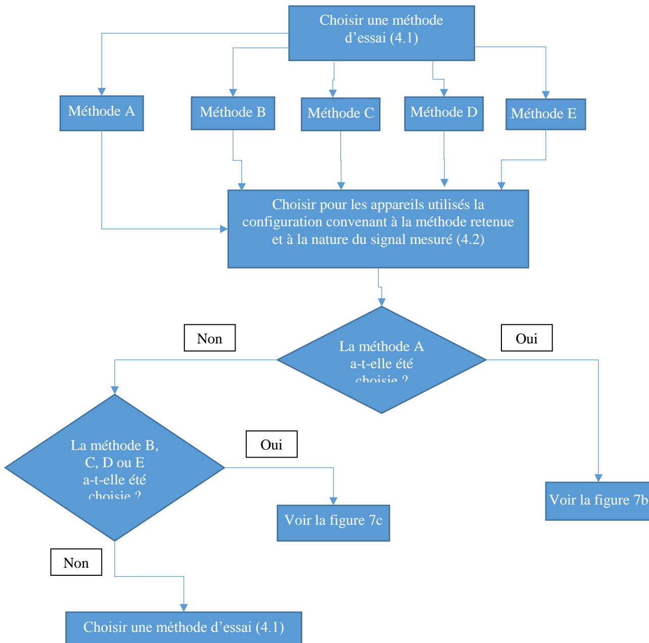
Figure 7a Méthodes d'essai pour la mesure du changement de fréquence
