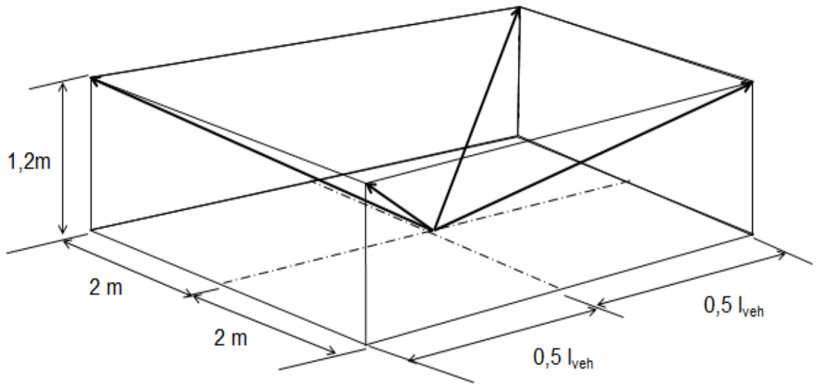
Figure 3 Espace minimal à respecter pour une chambre semi-anéchoïque
