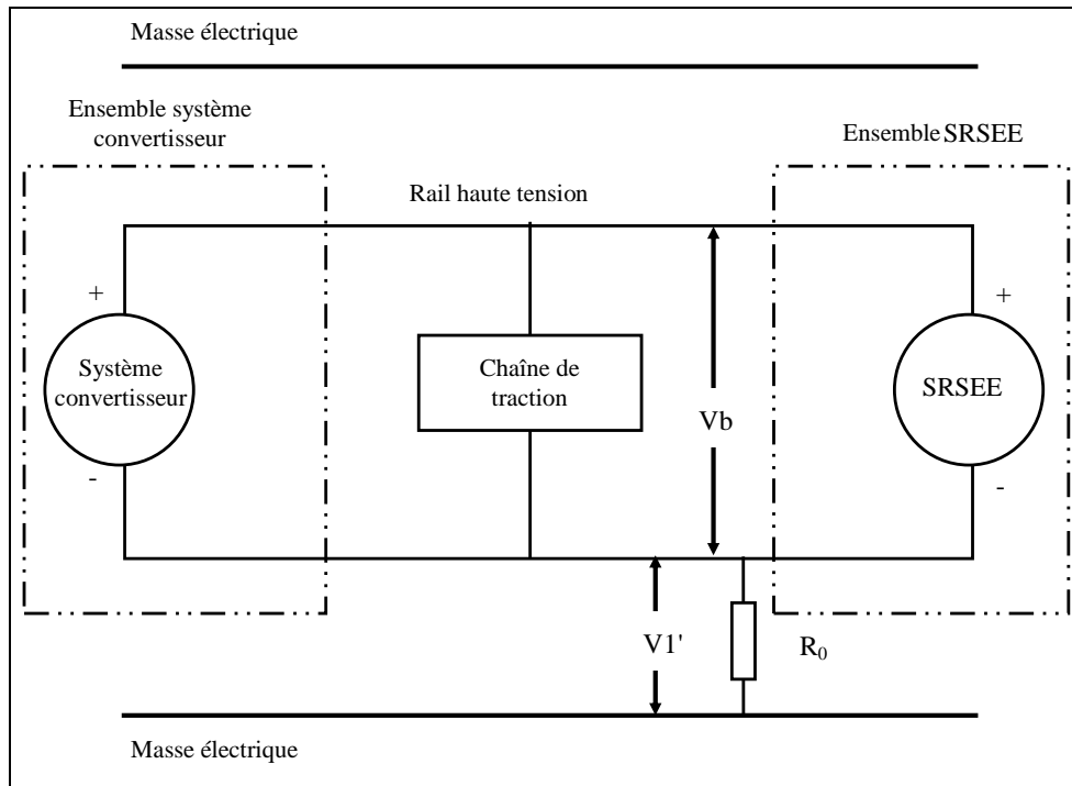
Figure 2 Mesure de V1'
