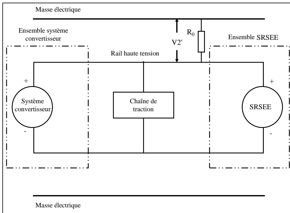
Figure 3 Mesure de V_2'
