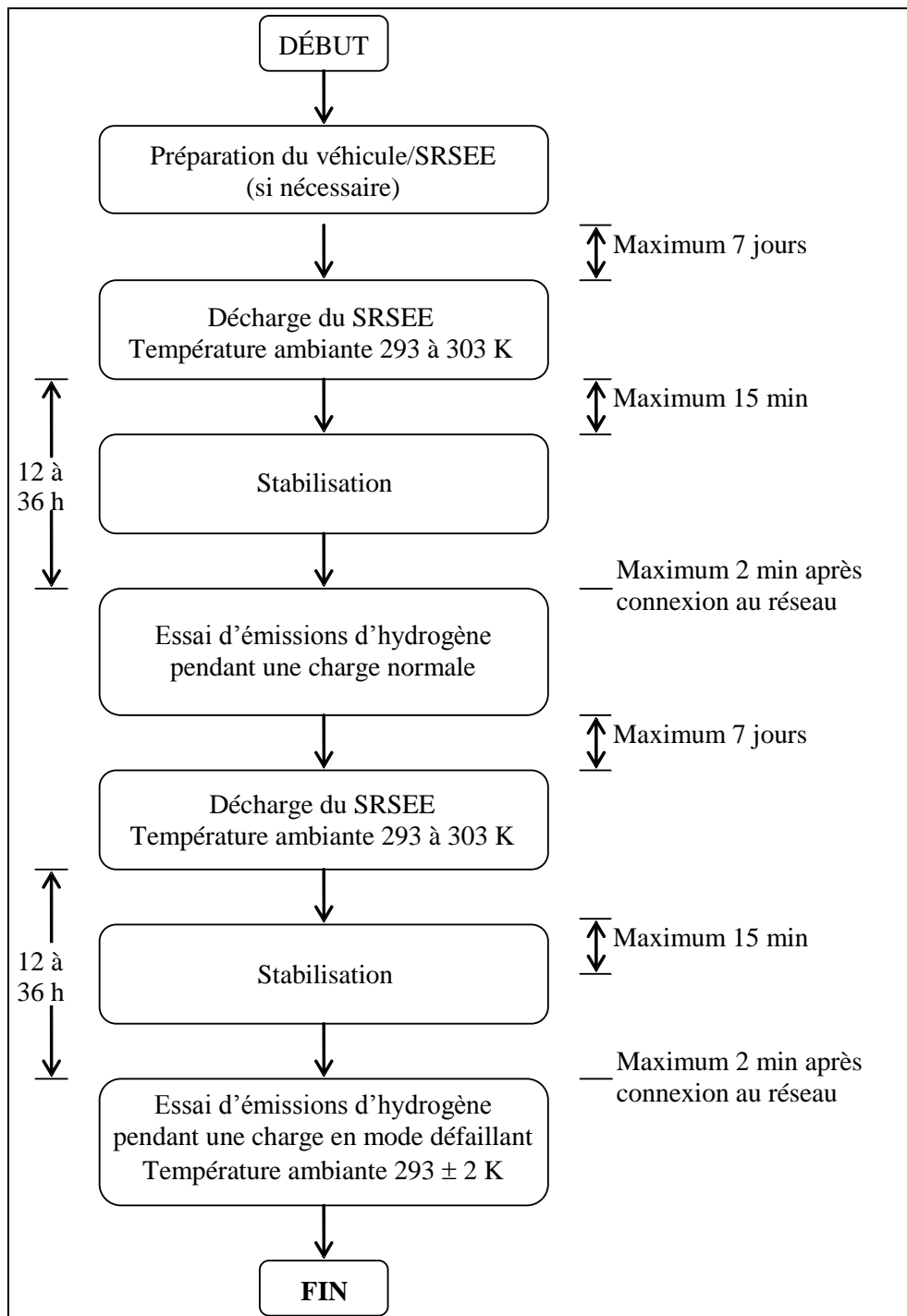
Figure 7.1 Détermination des émissions d'hydrogène pendant les opérations de charge du SRSEE
