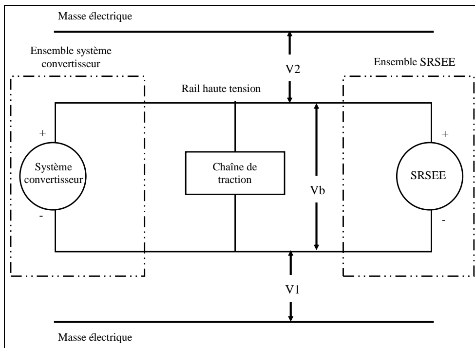
Figure 1 Mesure de V_b , V_1 , V_2
