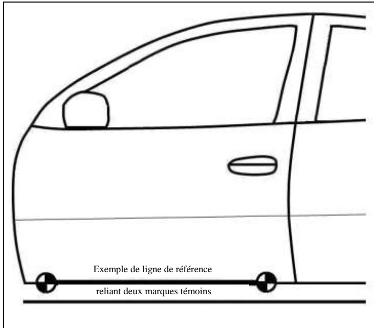
Figure 9-1 Exemple de ligne de référence reliant deux marques témoins sur le seuil de la porte avant gauche
