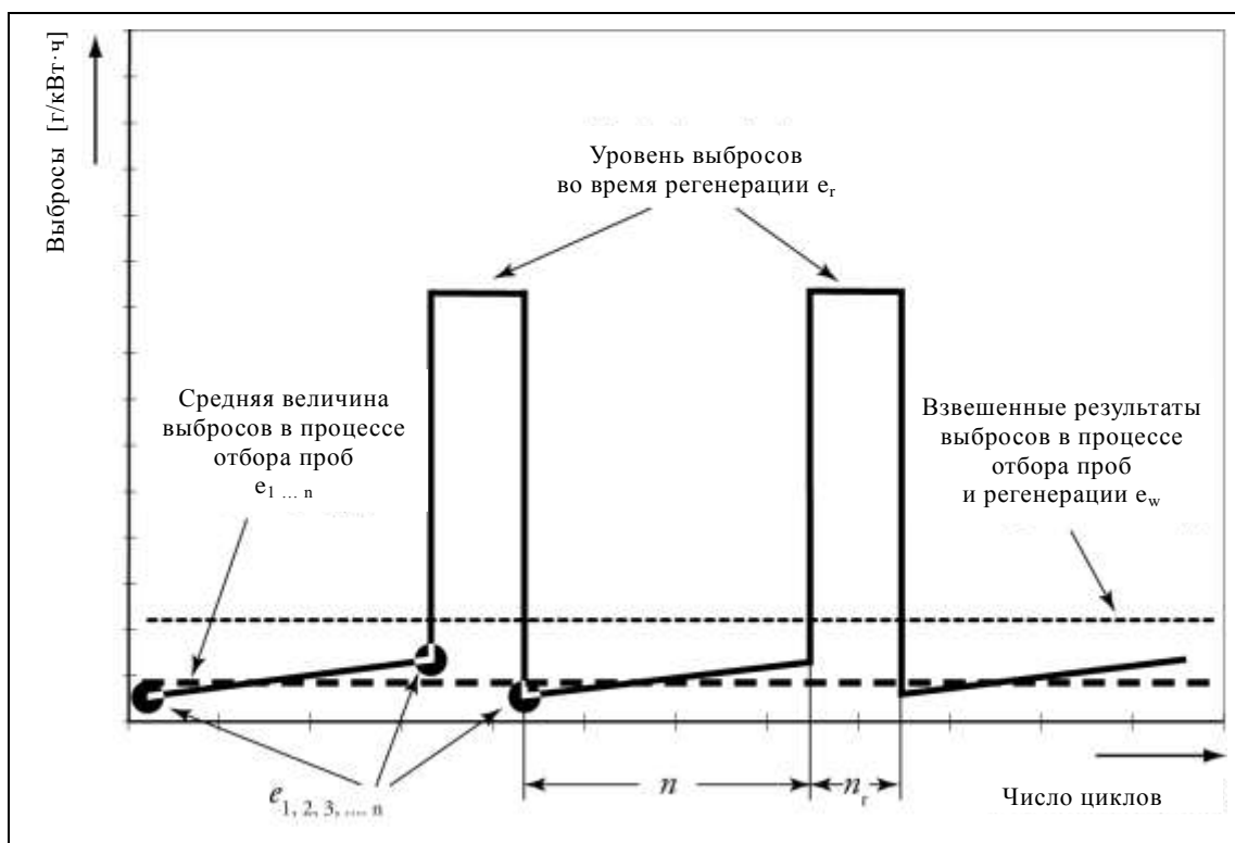
Рис. 1 Схема периодической регенерации
