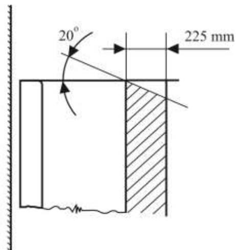
Longitudinal seat
