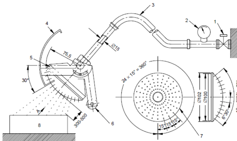
Dimensions en millimètres Vision depuis le point de vue indiquée par la flèche A (cache retiré) IEC 927/01
