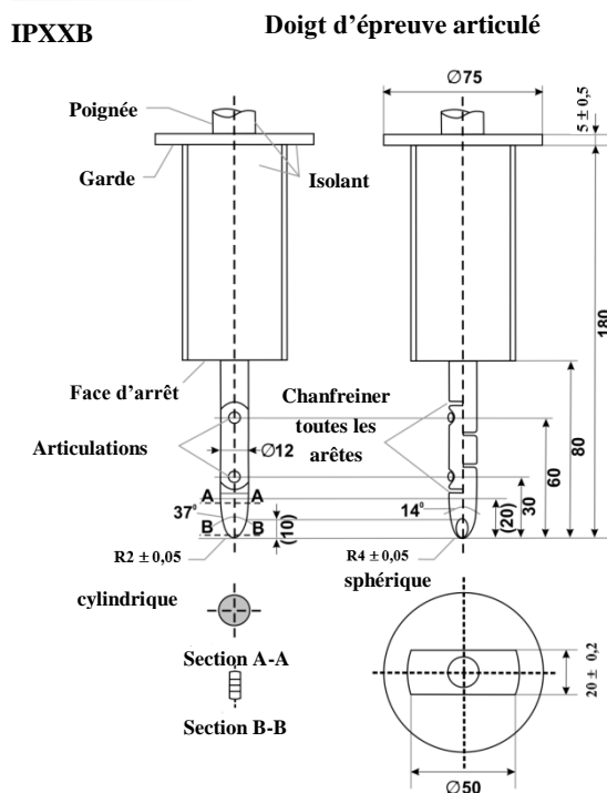
Figure 3 Doigt d'épreuve articulé Calibre d'accessibilité (dimensions en mm)
