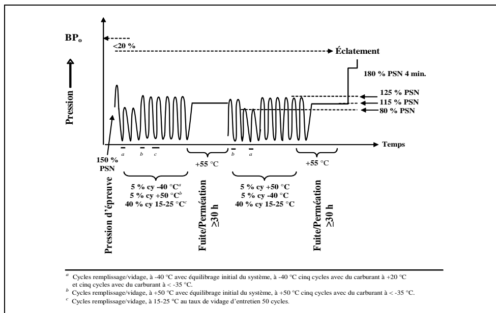
Figure 3 Essai de vérification des caractéristiques attendues en utilisation sur route (essais pneumatiques/hydrauliques)
