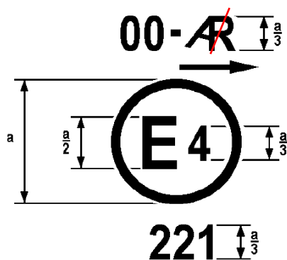
Рис. 1 Маркировка для одиночных огней
