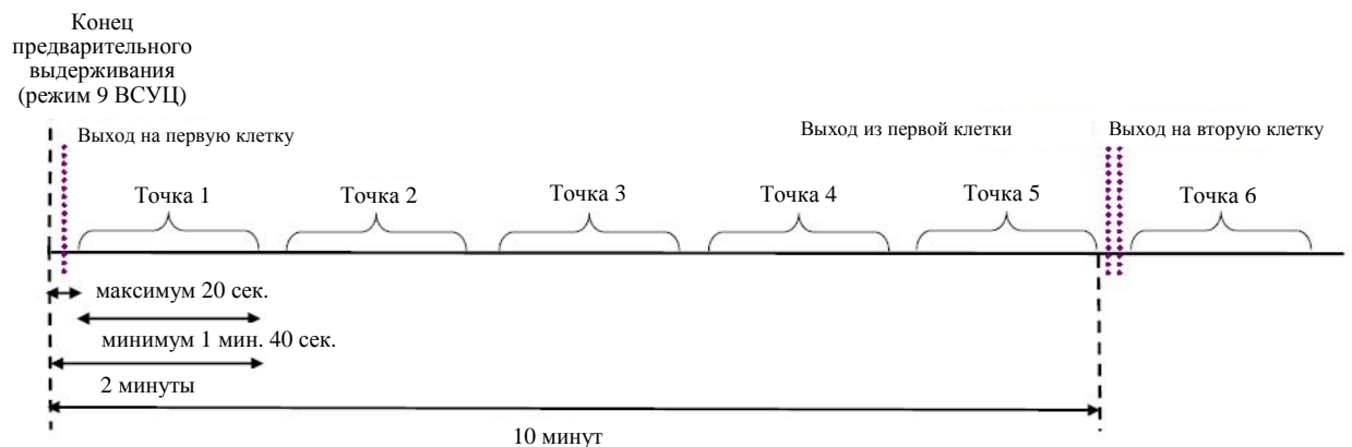
Рис. 4: Схематический пример начального этапа испытательного цикла ВСУЦ
