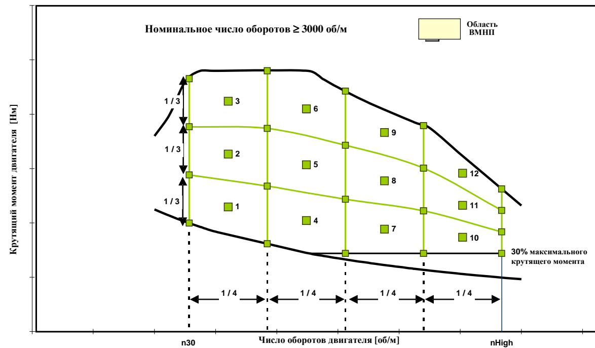
Рис. 5 и 6: Сетки испытательного цикла ВСУЦ
