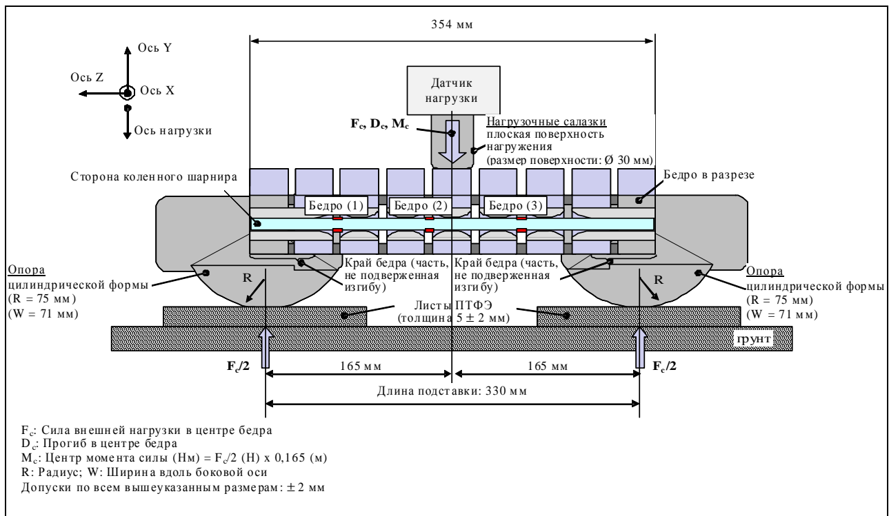
Рис. 24 Ударный элемент в виде гибкой модели нижней части ноги: испытательная установка для проведения испытания бедра при статических сертификационных испытаниях (см. пункт 8.1.1.4)
