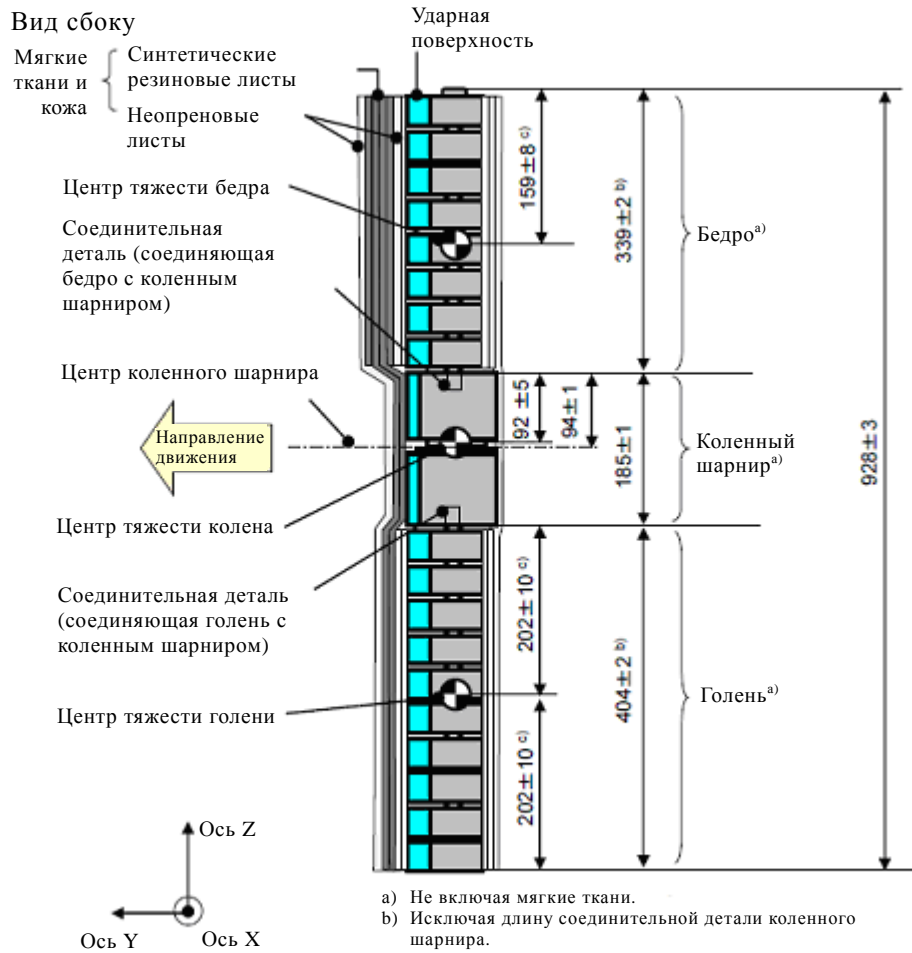
"Рис. 12 Ударный элемент в виде гибкой модели нижней части ноги: размеры и участки, на которых расположены центры тяжести бедра, коленного шарнира и голени (вид сбоку)
