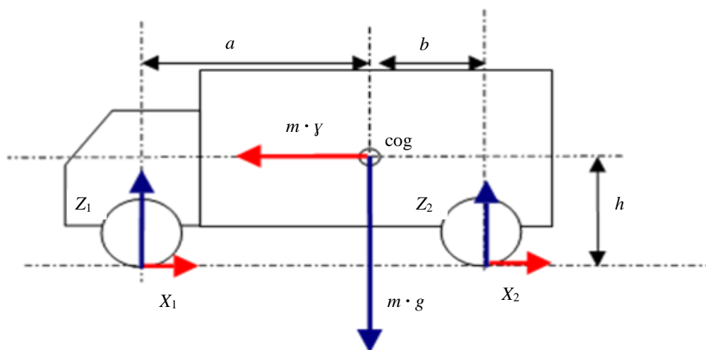
Рис. 1 Схематическое разъяснение, касающееся коэффициента сцепления шины
