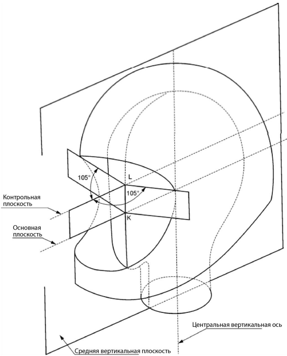
Рис. 2С Периферийный обзор – горизонтальное поле
