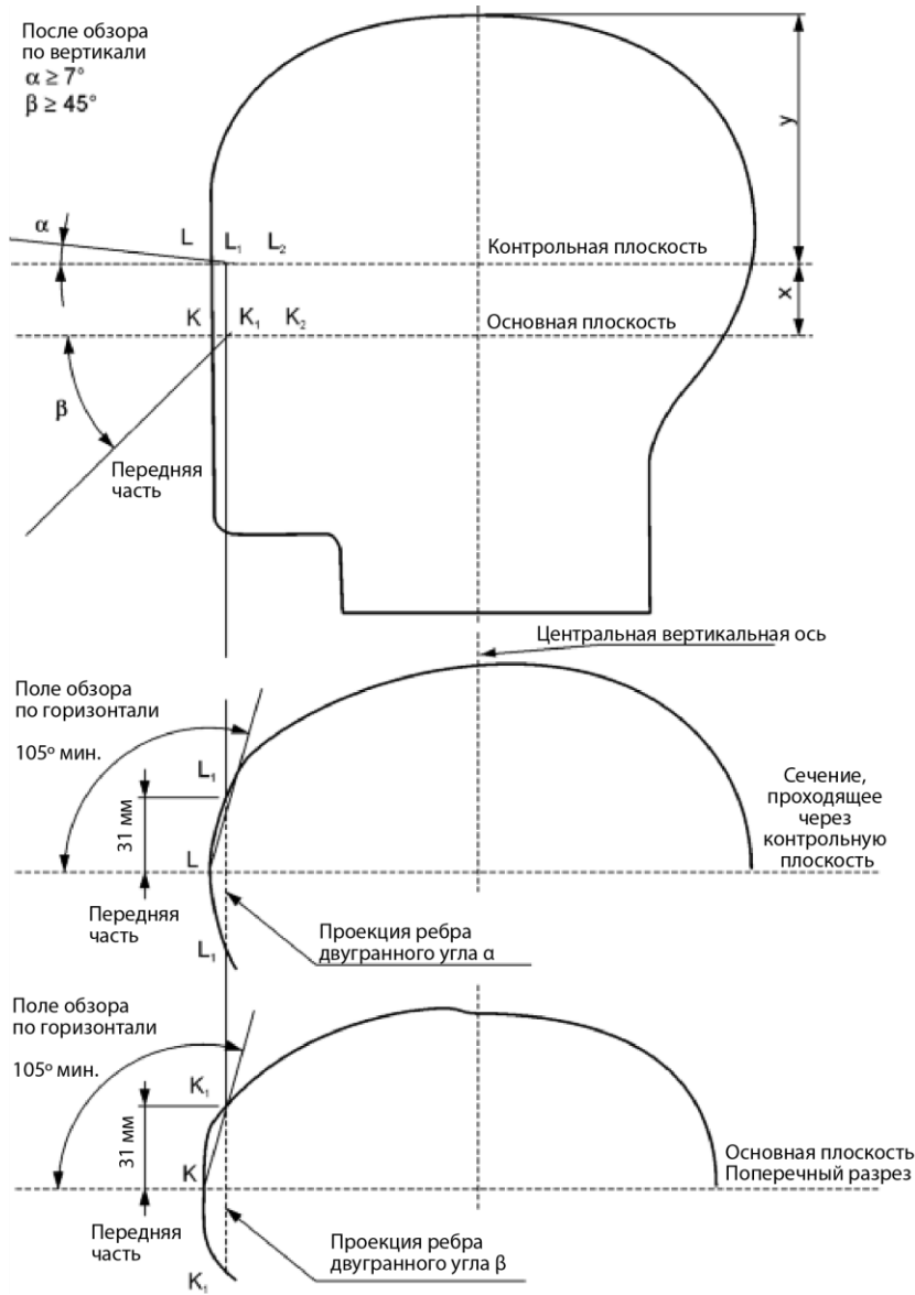
Рис. 2А Периферийный обзор
