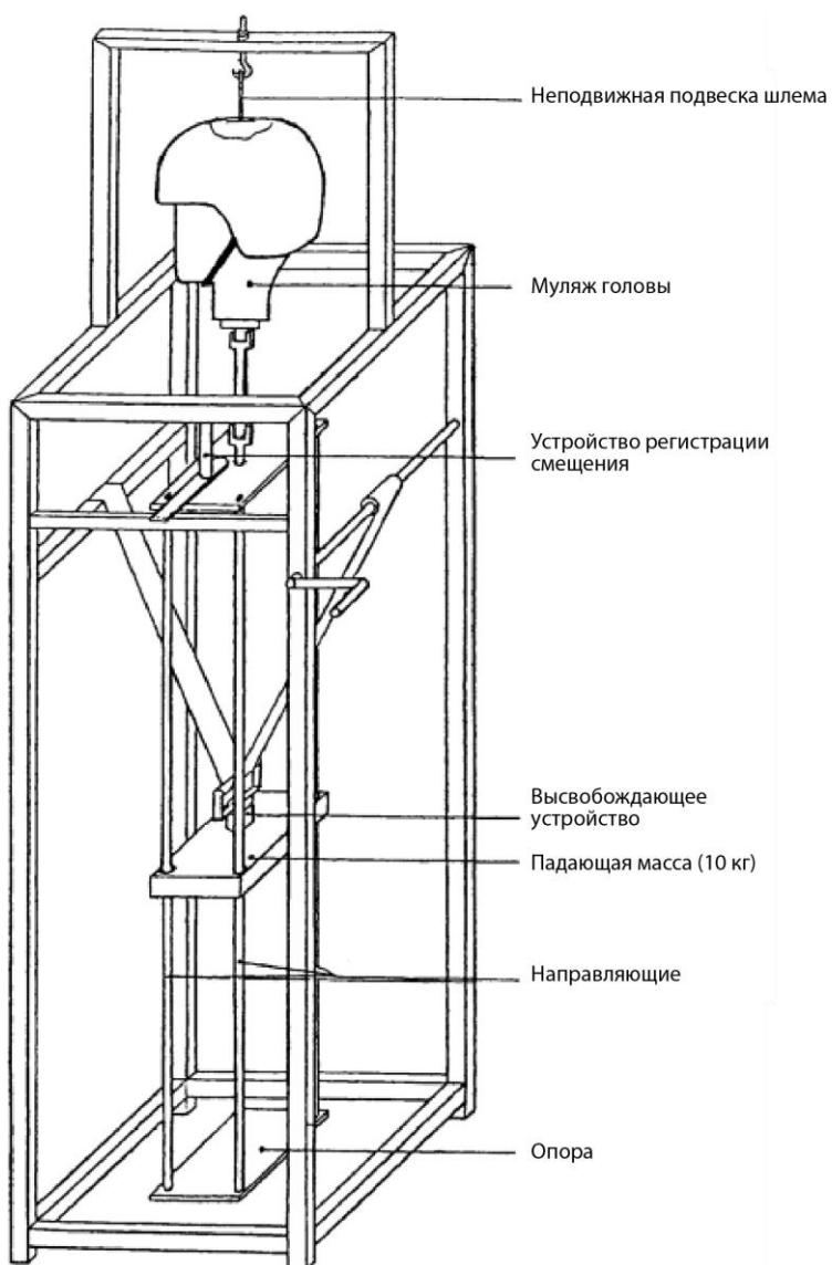
Рис. 2 Динамическое испытание удерживающей системы
