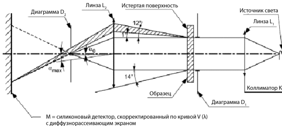
Рис. 2 Кольцевая диафрагма D 2
