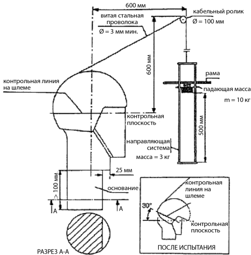
Рис. 3 Устройство для испытания на удержание
