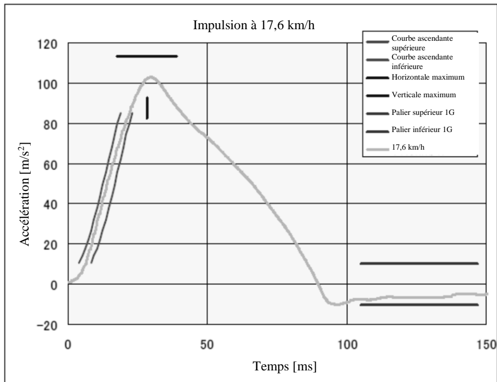
Figure 14-1 Courbe accélération/temps et tolérance admise de la courbe pour le montage d'essai conforme à la section 4.2 (l'accélération recherchée, le temps étant exprimé en millisecondes, doit être conforme à la valeur indiquée dans le tableau 14-2.)
