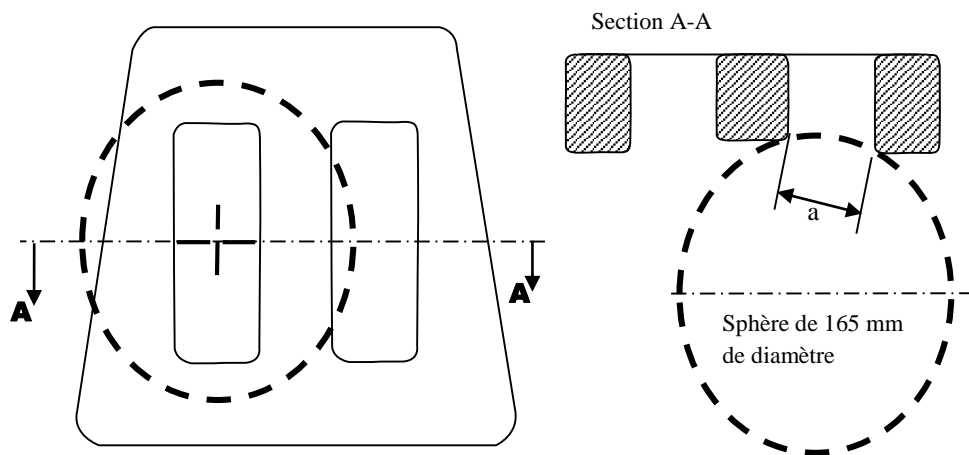
Figure 8-2 Mesure d'une discontinuité horizontale "a".
