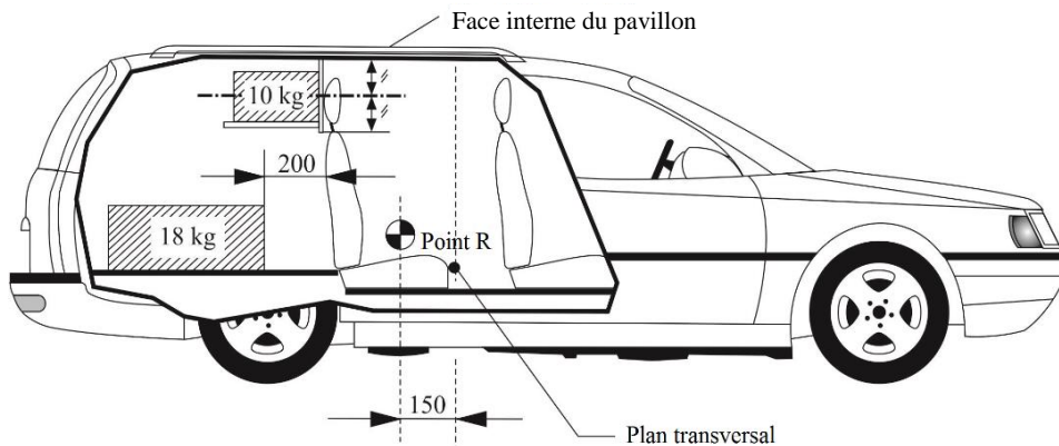
Figure 9-2 Essai d'un dispositif de cloisonnement situé au-dessus des appuie-tête
