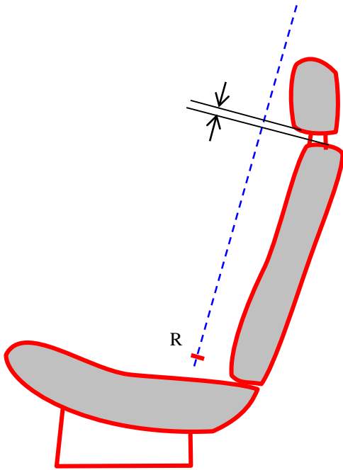
Figure 8-3 Espace entre l'appui-tête et le sommet du dossier du siège
