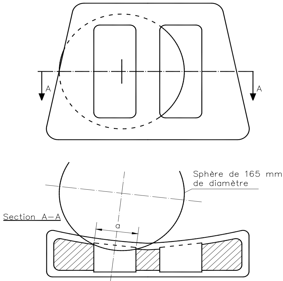
Figure 2 Exemple de discontinuité verticale
