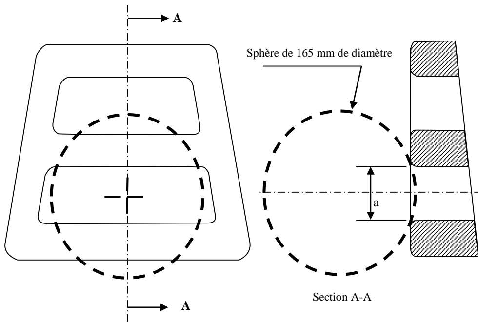
Figure 8-1+ Mesure d'une discontinuité verticale "a". Exemple de discontinuité horizontale
