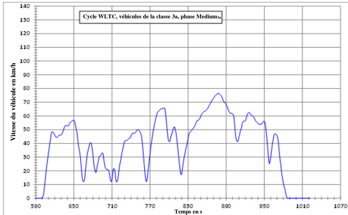
Figure A1/8 Cycle WLTC, véhicules de la classe 3a, phase Medium 3a
