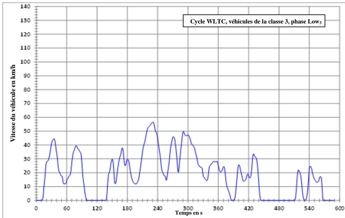
Figure A1/7 Cycle WLTC, véhicules de la classe 3, phase Low 3
