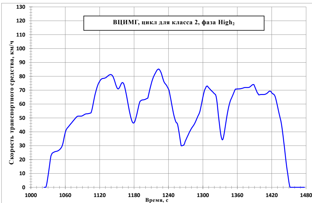
Рис. А1/5 ВЦИМГ, цикл применительно к классу 2, фаза High 2
