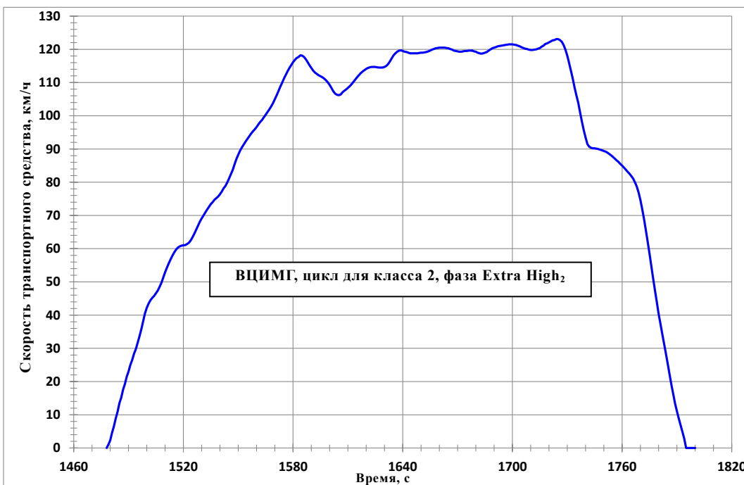
Рис. А1/6 ВЦИМГ, цикл применительно к классу 2, фаза Extra High 2
