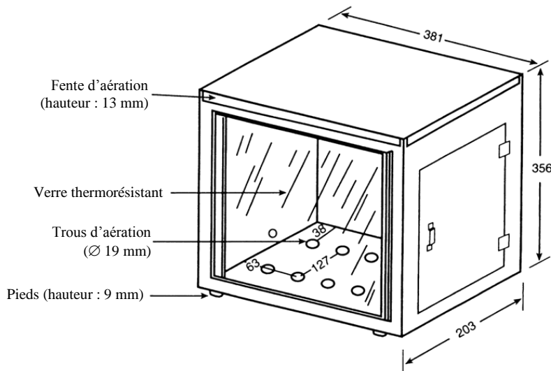
Figure 2 Toutes les dimensions sont en millimètres (mm)
