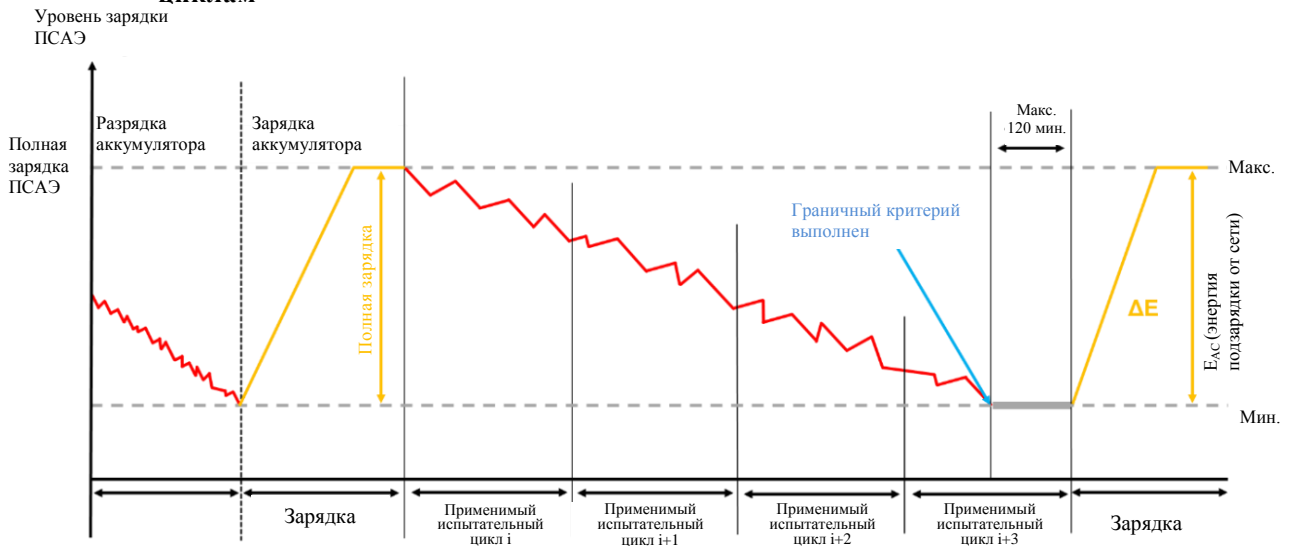
Рис. А8.App1/6 Последовательность испытания ПЭМ с прогоном по последовательным циклам
