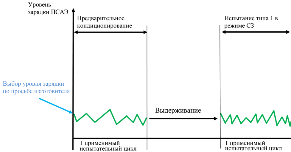
Рис. А8.App1/5 ГЭМ-БЗУ и ГТСТЭ-БЗУ, испытание типа 1 в режиме сохранения заряда
