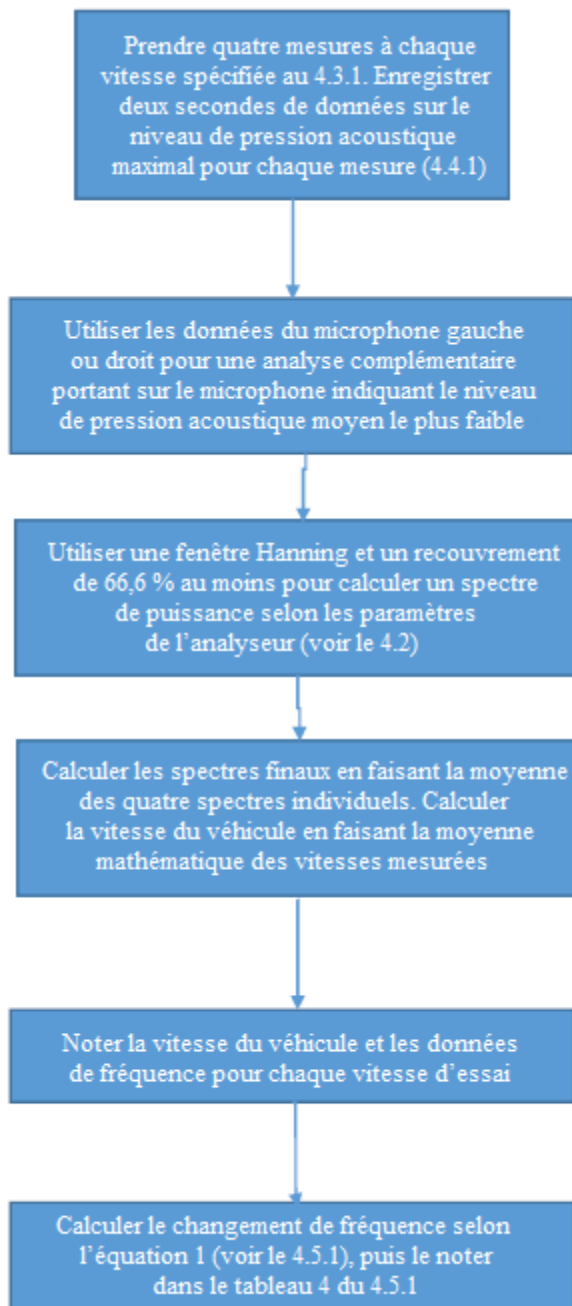
Figure 7b Procédure d'essai pour la mesure du changement de fréquence – méthode A
