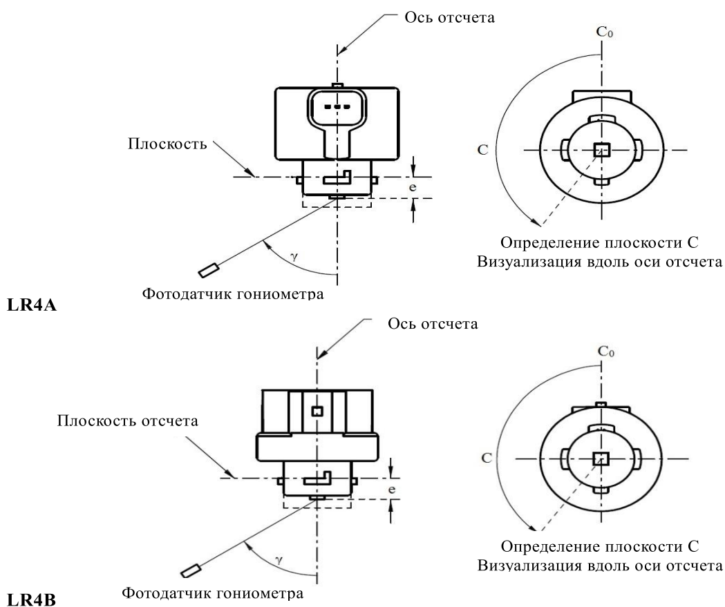
Рис. 3* Схема измерения распределения силы света
