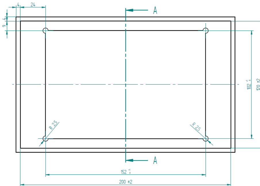
Figure 1 Vue de dessus de la boîte (dimensions en mm)
