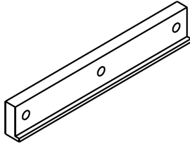
Figure 4 Vue en trois dimensions du porte-lame (après insertion de la lame dans la plaque d'entretoise, la contre-plaque est attachée et fixée avec trois vis)
