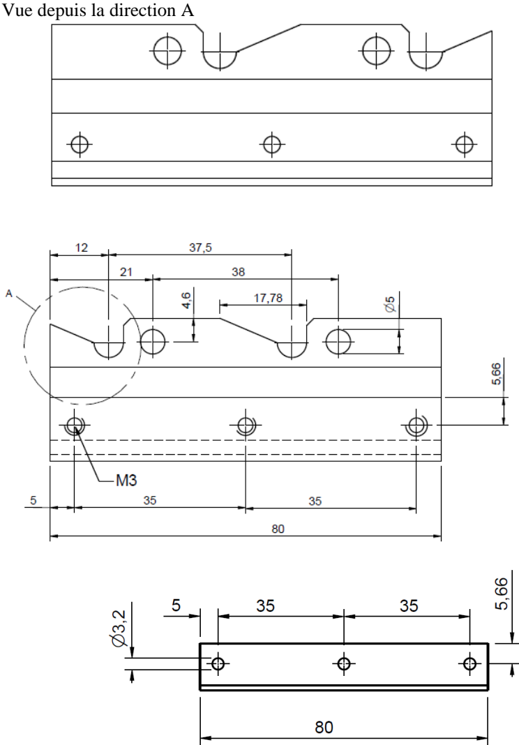
Figure 3 Détails concernant la zone A dans la figure 2
