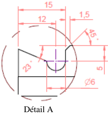
Figure 3 Détails concernant la zone A dans la figure 2
