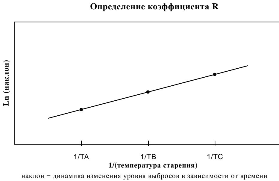
Рис. А9.Аpp1/4 Определение коэффициента R
