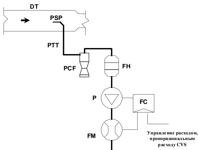
Рис. A4a.App4/12 Система отбора проб частиц
