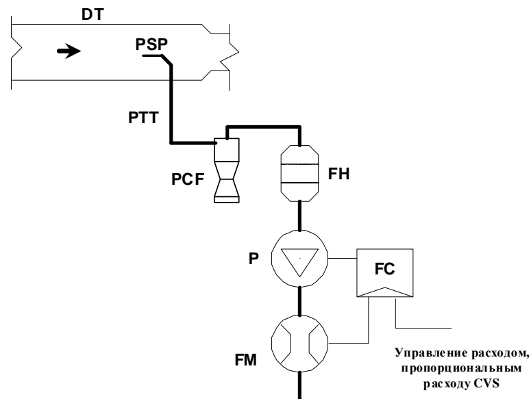
Рис. А4а. App4/12 Система отбора проб частиц
