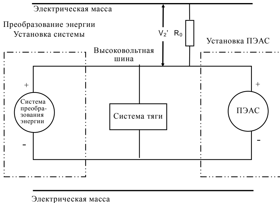
Рисунок 4 Измерение V_2'
