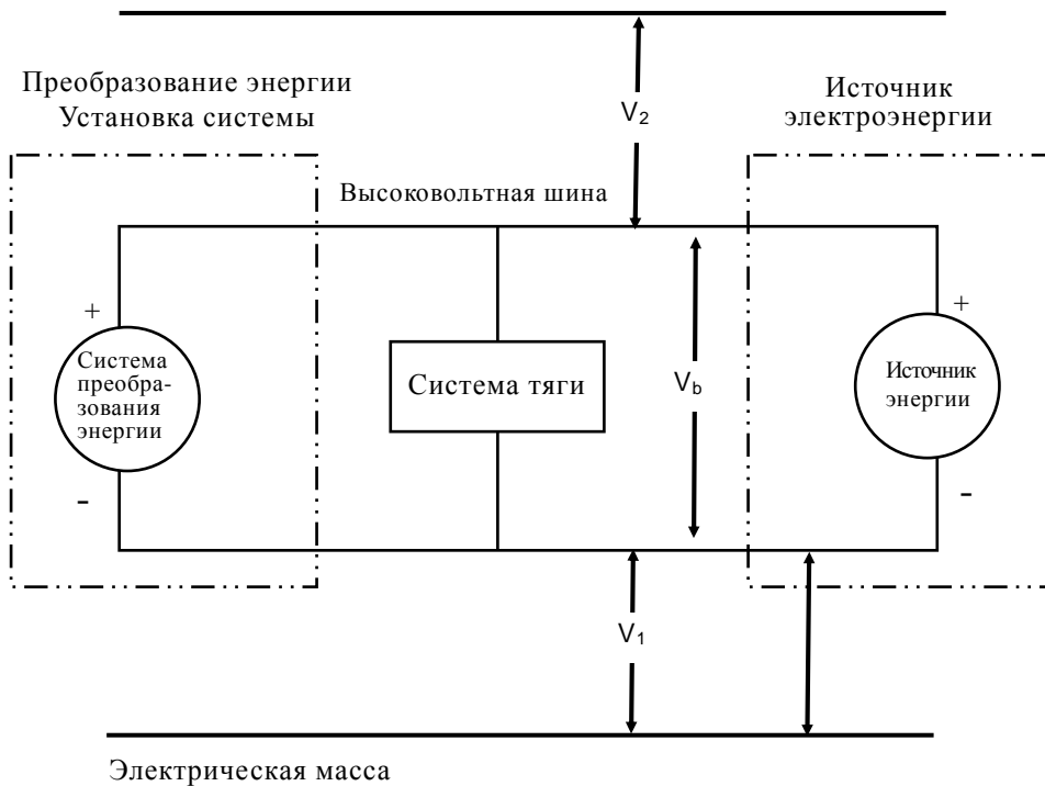
Рисунок 1 Измерение V_b , V_1 , V_2
