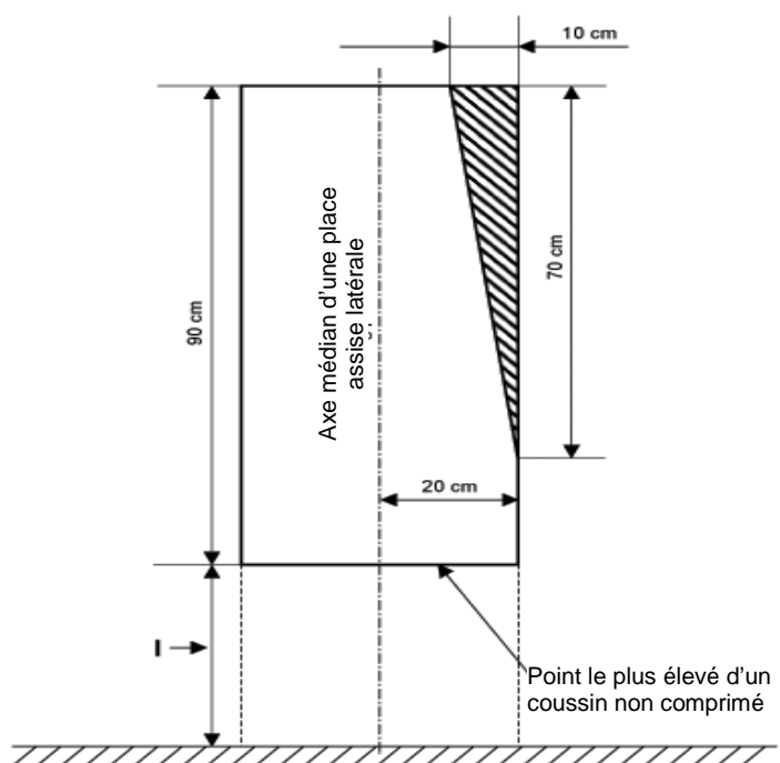
« Figure 7 Intrusion autorisée d'un élément de structure (voir par. 5.7.8.1.3.2)
