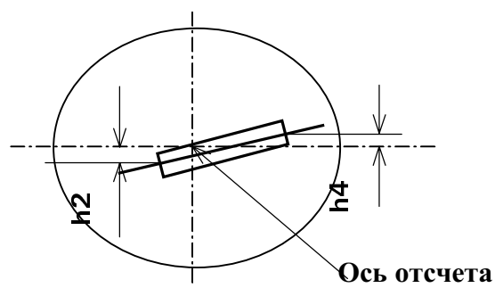
Рис. 3. Расположение и размеры нити накала
