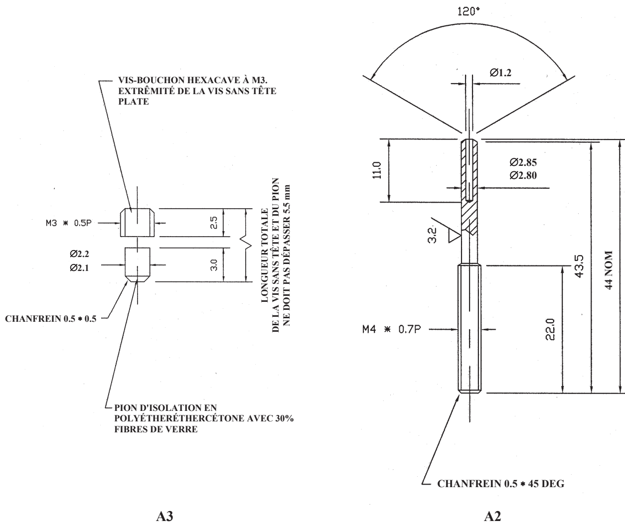
Figure A7.5 : PARTIES A3 ET A2
