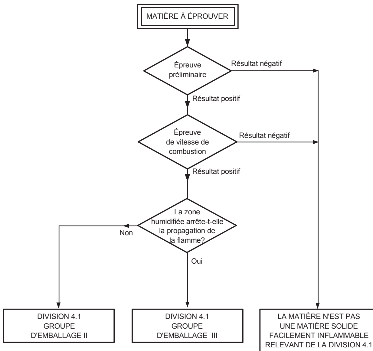
FIGURE 33.2.1.3: DIAGRAMME DE DÉCISION POUR L'AFFECTION DES MATIÈRES SOLIDES FACILEMENT INFLAMMABLES (à l'exception des poudres métalliques) À LA DIVISION 4.1
