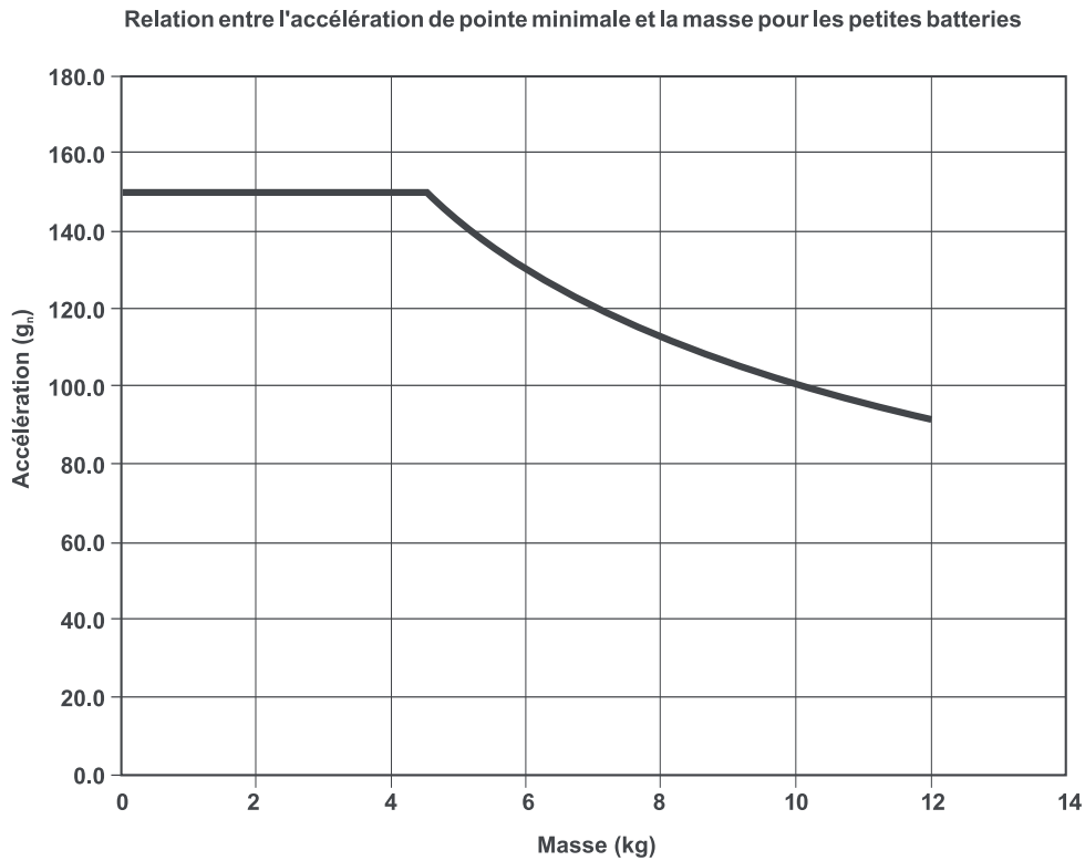
Figure 38.3.4.1: RELATION ENTRE L'ACCELERATION DE POINTE MINIMALE ET LA MASSE POUR LES PETITES BATTERIES (inférieure ou égale à 12,0 kg)
