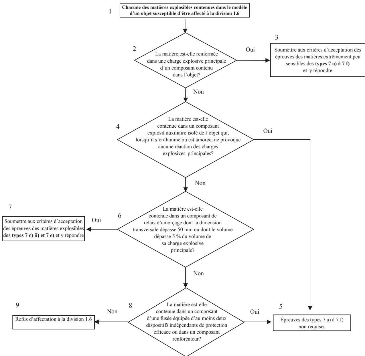
Figure 10.5: PROCEDURE VISANT A DETERMINER LES EPREUVES QUE DOIVENT SUBIR LES MATIERES CONTENUES DANS UN OBJET EN VUE DE SON AFFECTATION A LA DIVISION 1.6
