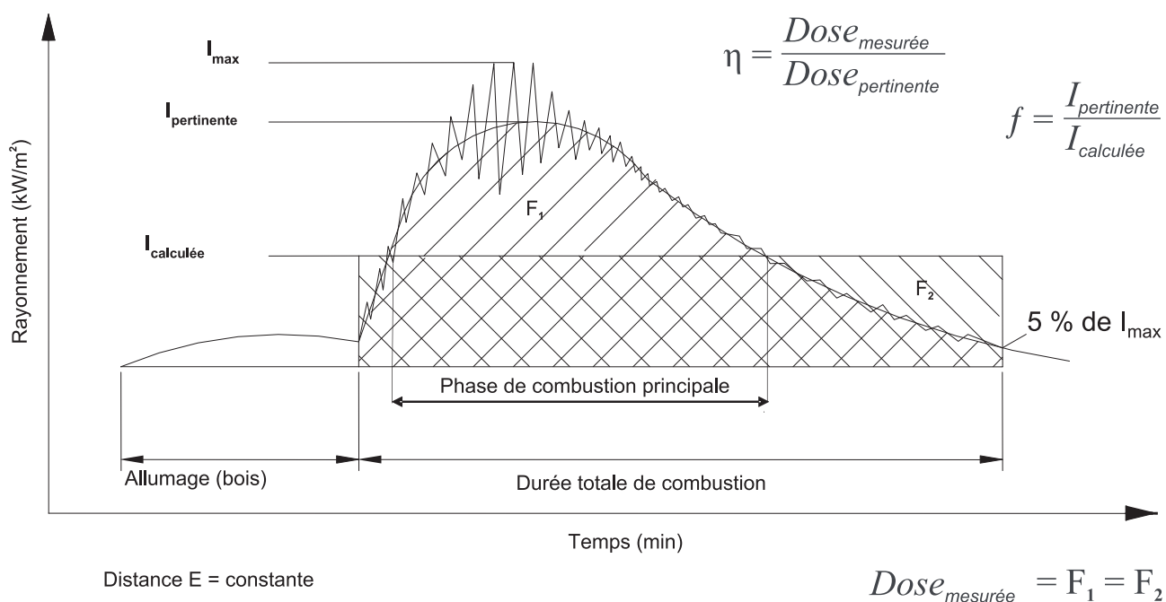
Figure 51.4.1: MESURE DU RAYONNEMENT EN FONCTION DU TEMPS
