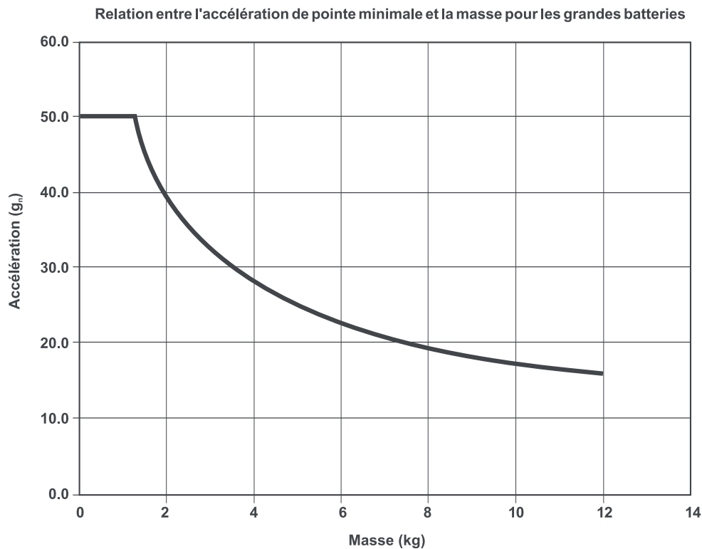
Figure 38.3.4.2: RELATION ENTRE L'ACCELERATION DE POINTE MINIMALE ET LA MASSE POUR LES GRANDES BATTERIES (au-dessus de 12,0 kg)
