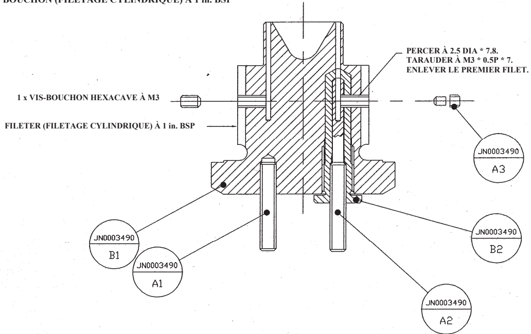
Figure A7.3 : ASSEMBLAGE
