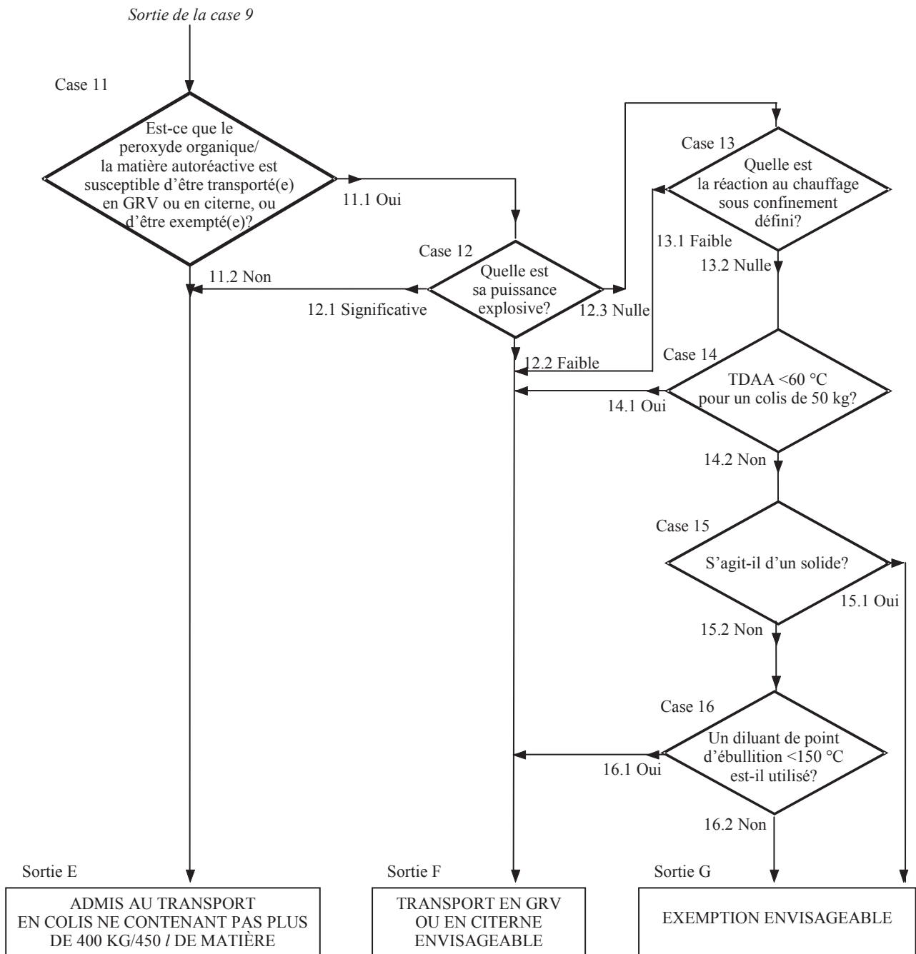
Figure 20.1 b): DIAGRAMME DE DÉCISION POUR LE CLASSEMENT DES MATIÈRES AUTORÉACTIVES ET DES PEROXYDES ORGANIQUES (suite)
