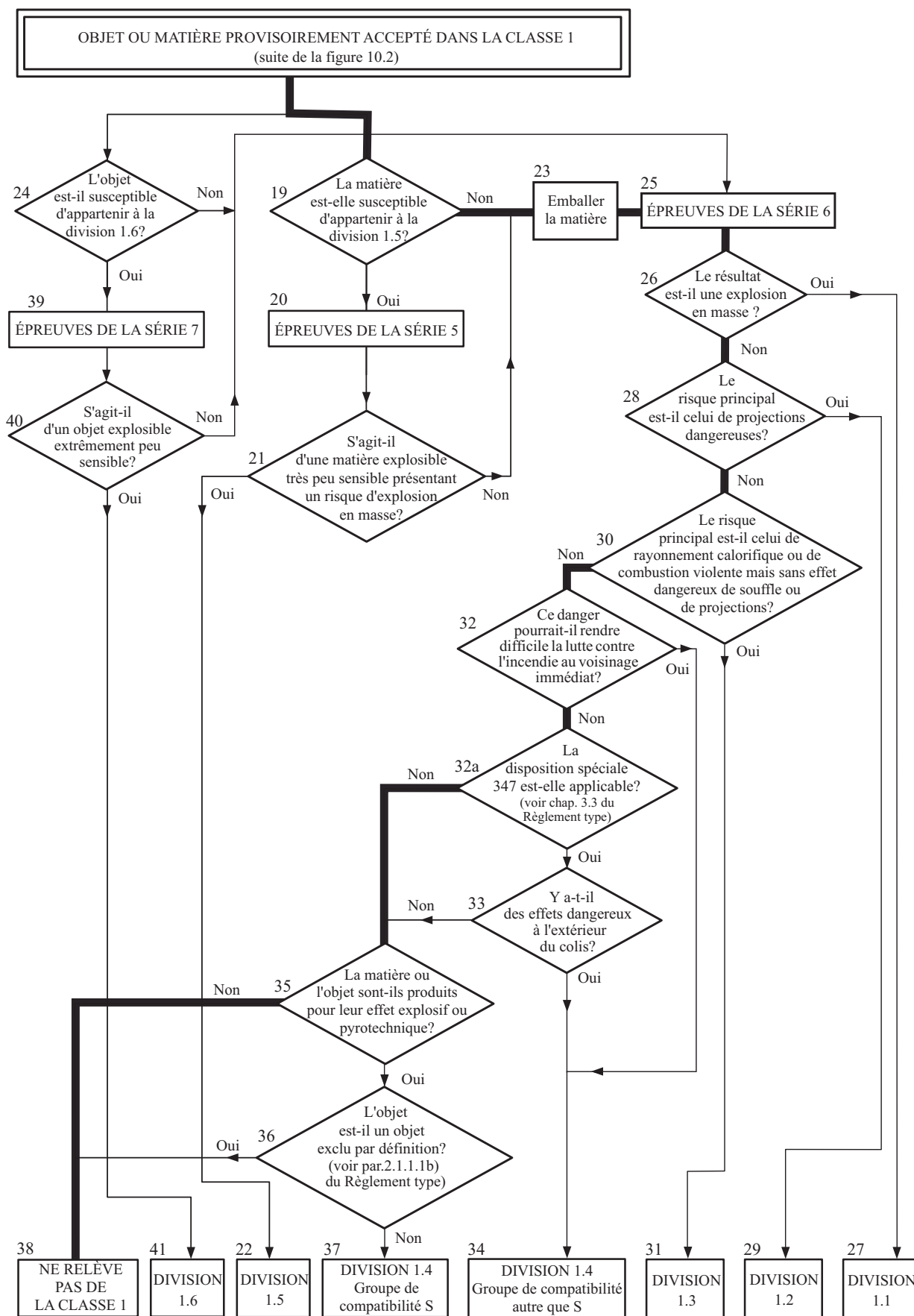
Figure 10.9: PROCÉDURE D'EXCLUSION DU TERT-BUTYLTRINITROXYLÈNE DE LA CLASSE 1
