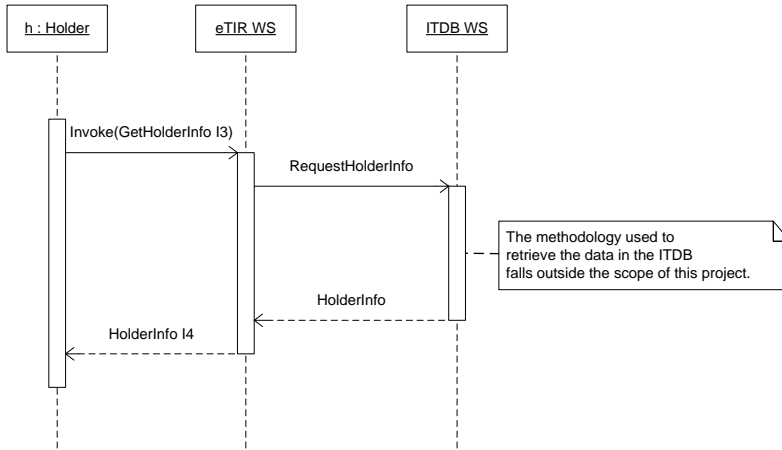
Диаграмма последовательности получения информации о держателе (только на английском языке)
