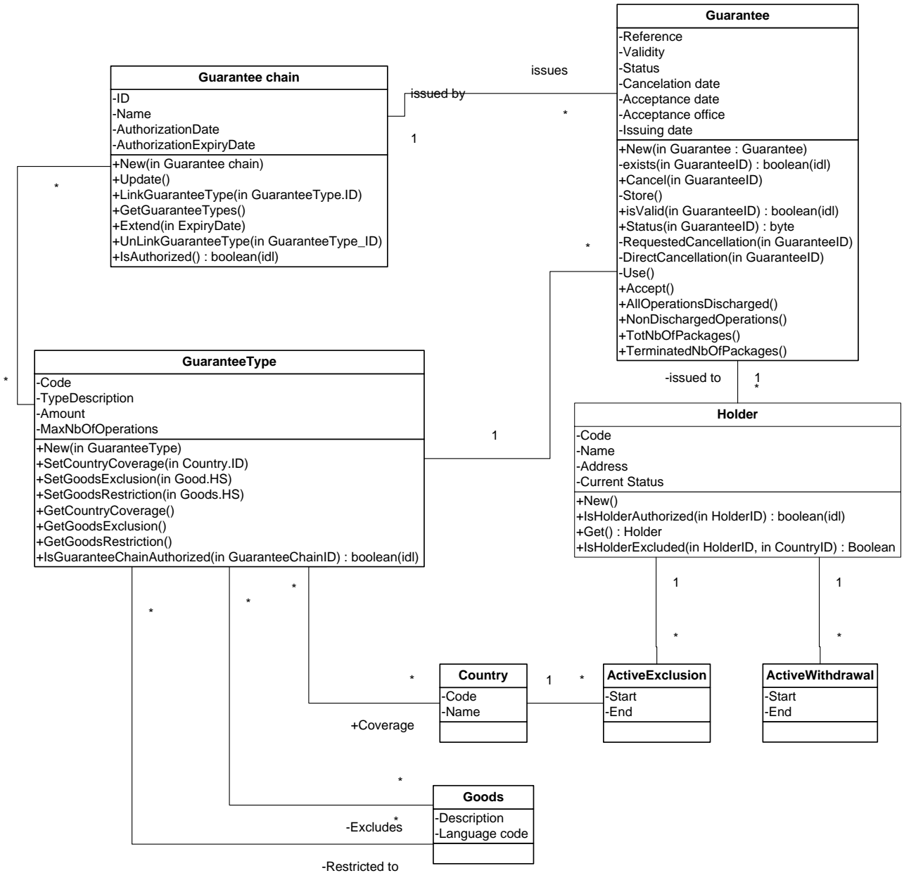
Рис. 3.16 (только на английском языке)
