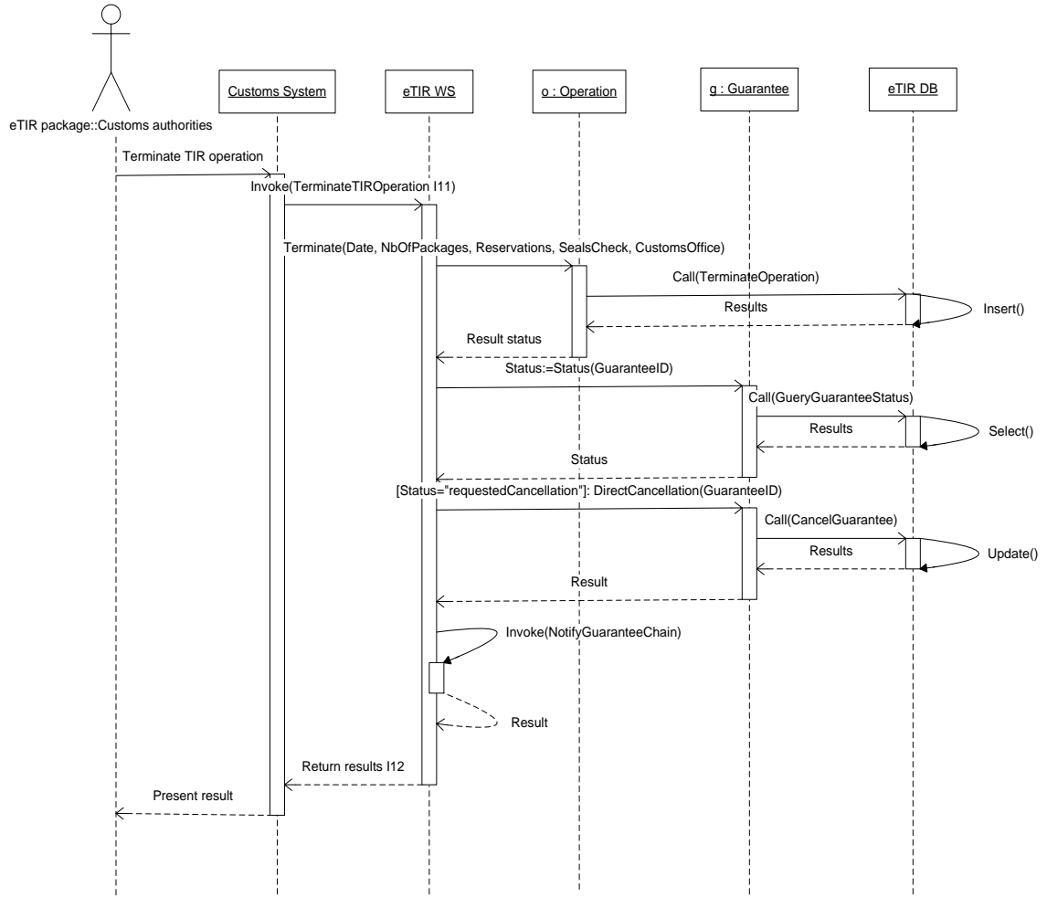
Рис. 3.11 Диаграмма последовательности прекращения операции МДП (только на английском языке)
