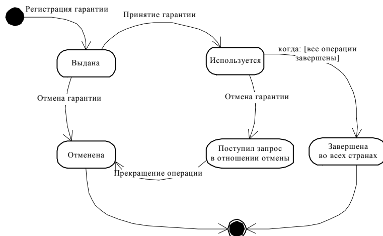
Рис. 2.3 Диаграмма статусов гарантии
