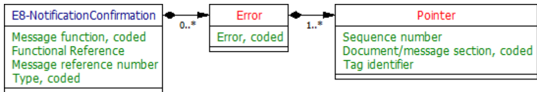
Рис. 3.26: (только на английском языке) Notification confirmation UML diagram
