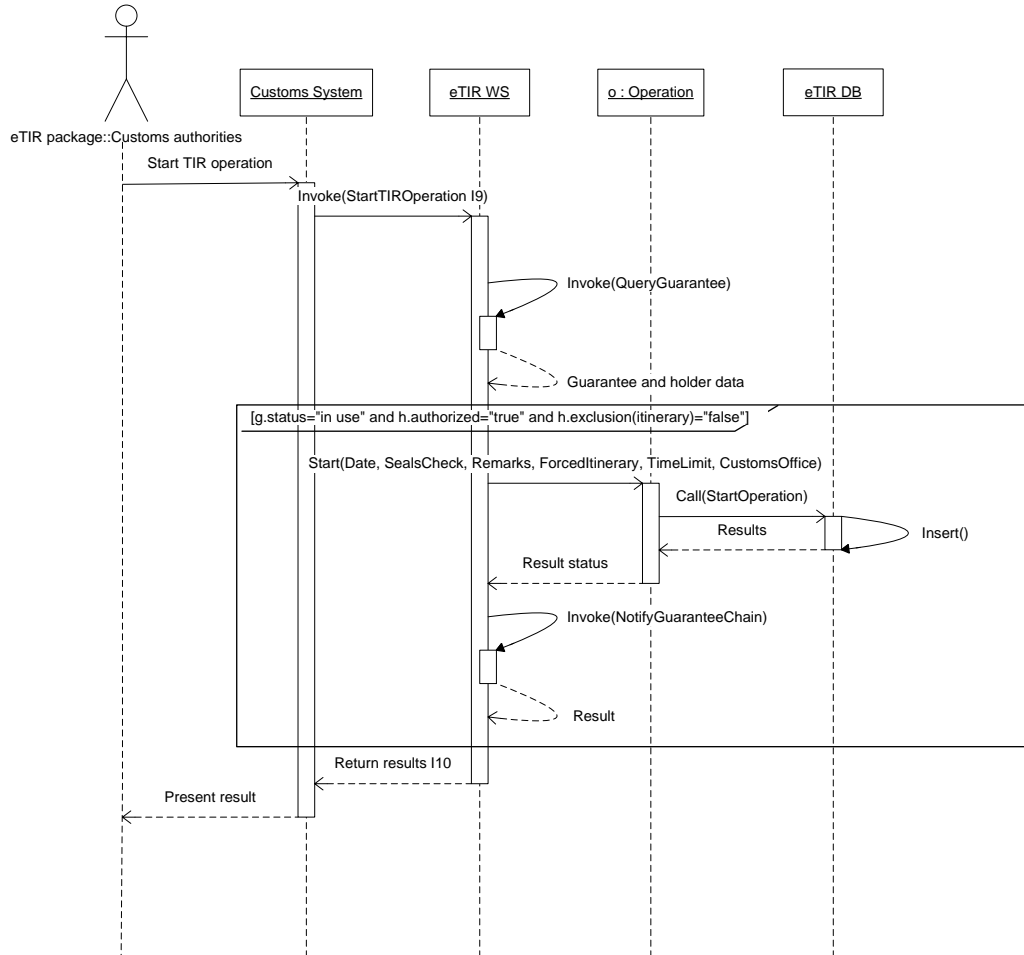
Рис. 3.10 Диаграмма последовательности начала операции МДП (только на английском языке)
