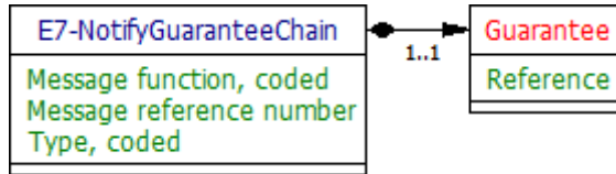
Рис. 3.25: (только на английском языке) Notify guarantee chain UML diagram
