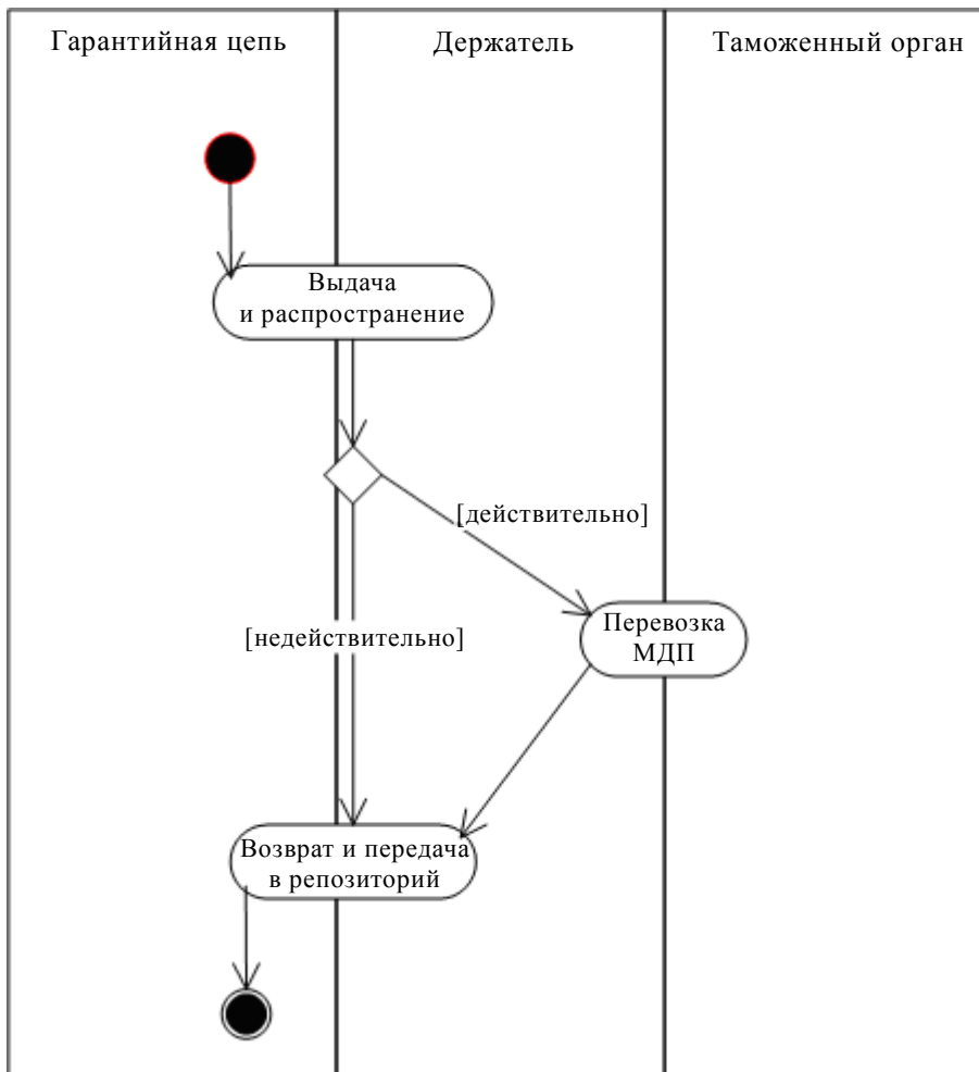
Диаграмма деятельности в рамках жизненного цикла книжки МДП
