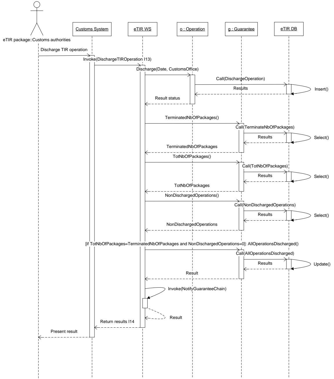
Рис. 3.12 Диаграмма последовательности завершения операции МДП (только на английском языке)
