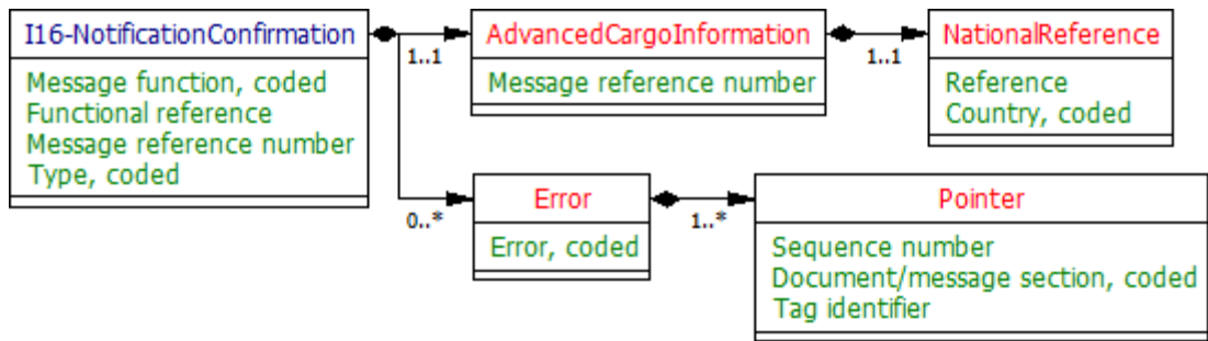
Рис. 3.44: (только на английском языке) Notification confirmation UML diagram
