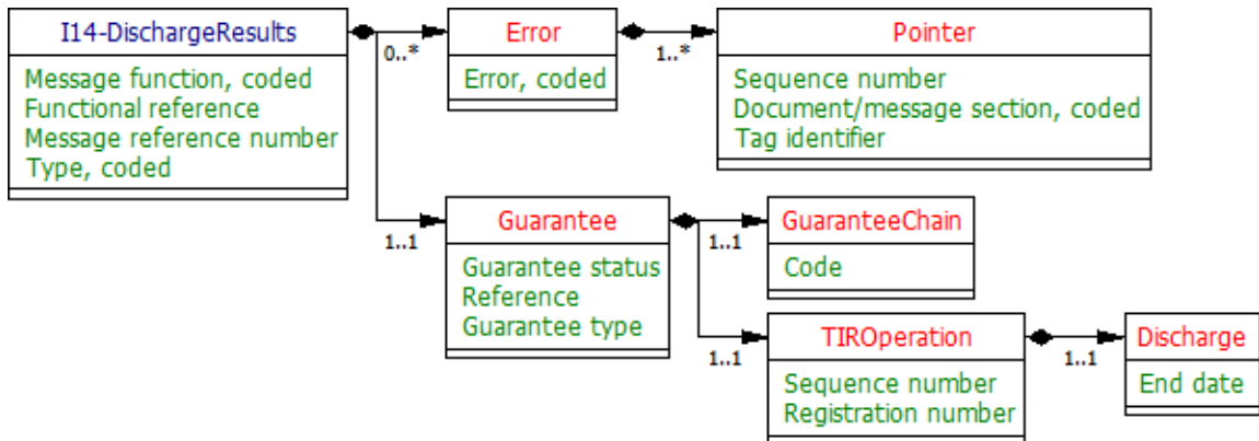
Рис. 3.42: (только на английском языке) Discharge results UML diagram
