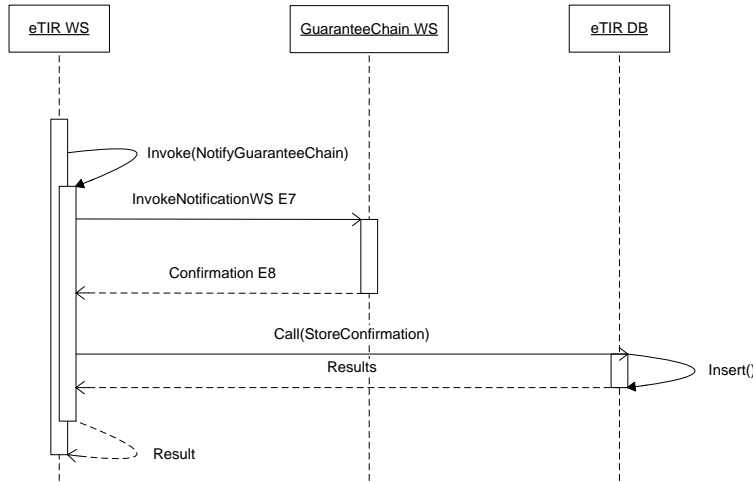
Рис. 3.13 Диаграмма последовательности уведомления гарантийной цепи (только на английском языке)
