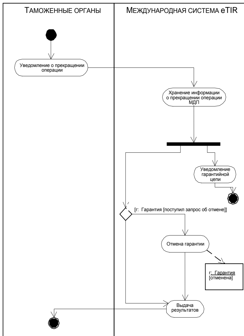
Диаграмма деятельности в случае прекращения операции МДП
