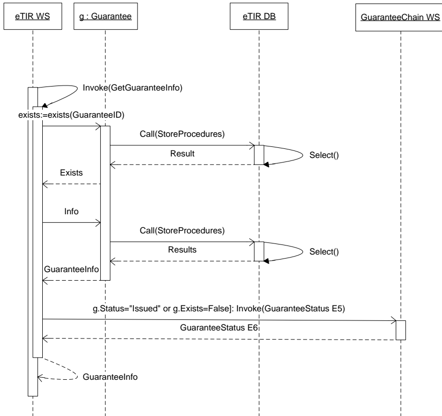
Диаграмма последовательности получения информации о гарантии (только на английском языке)
