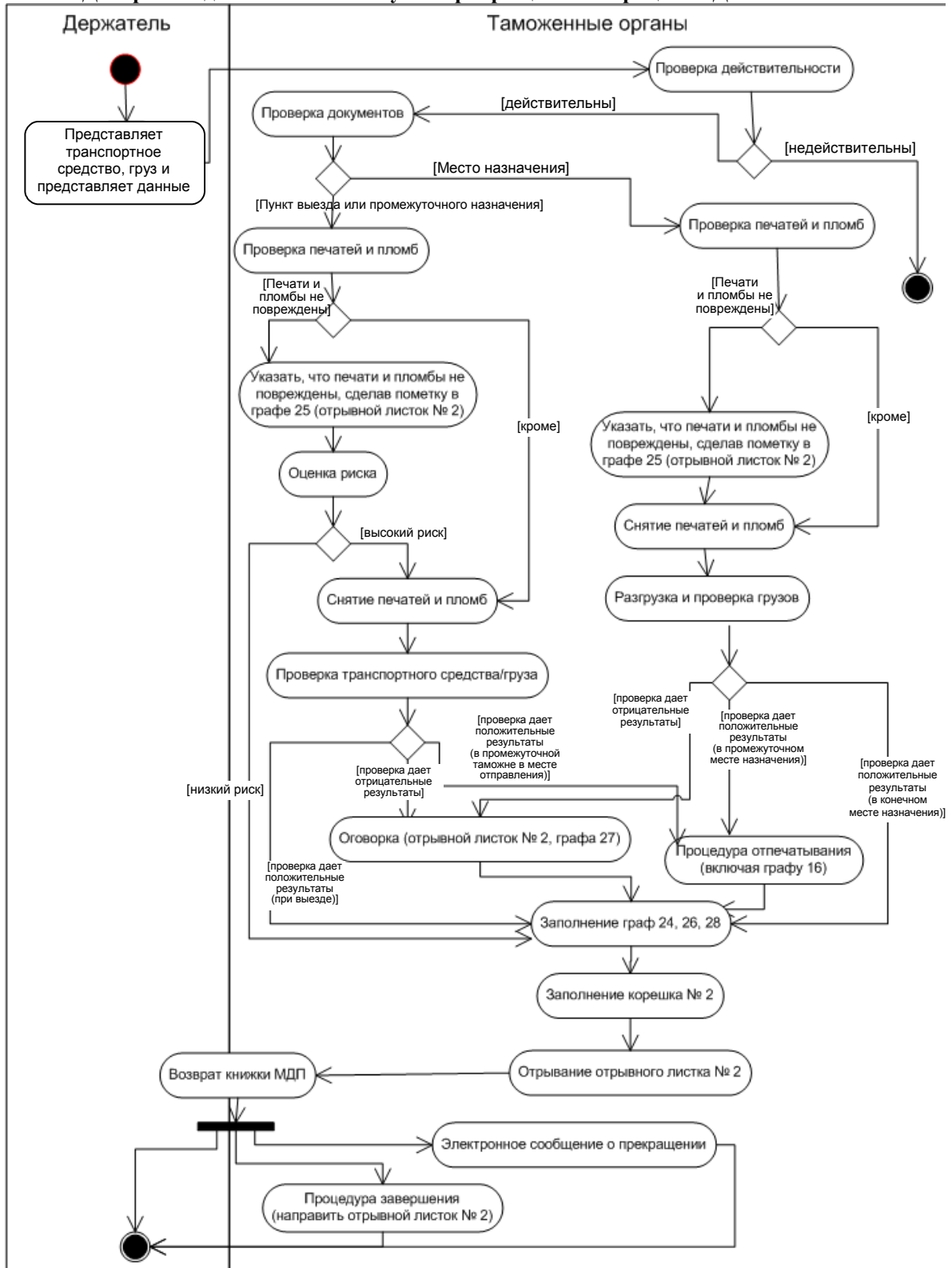
Диаграмма деятельности в случае прекращения операции МДП
