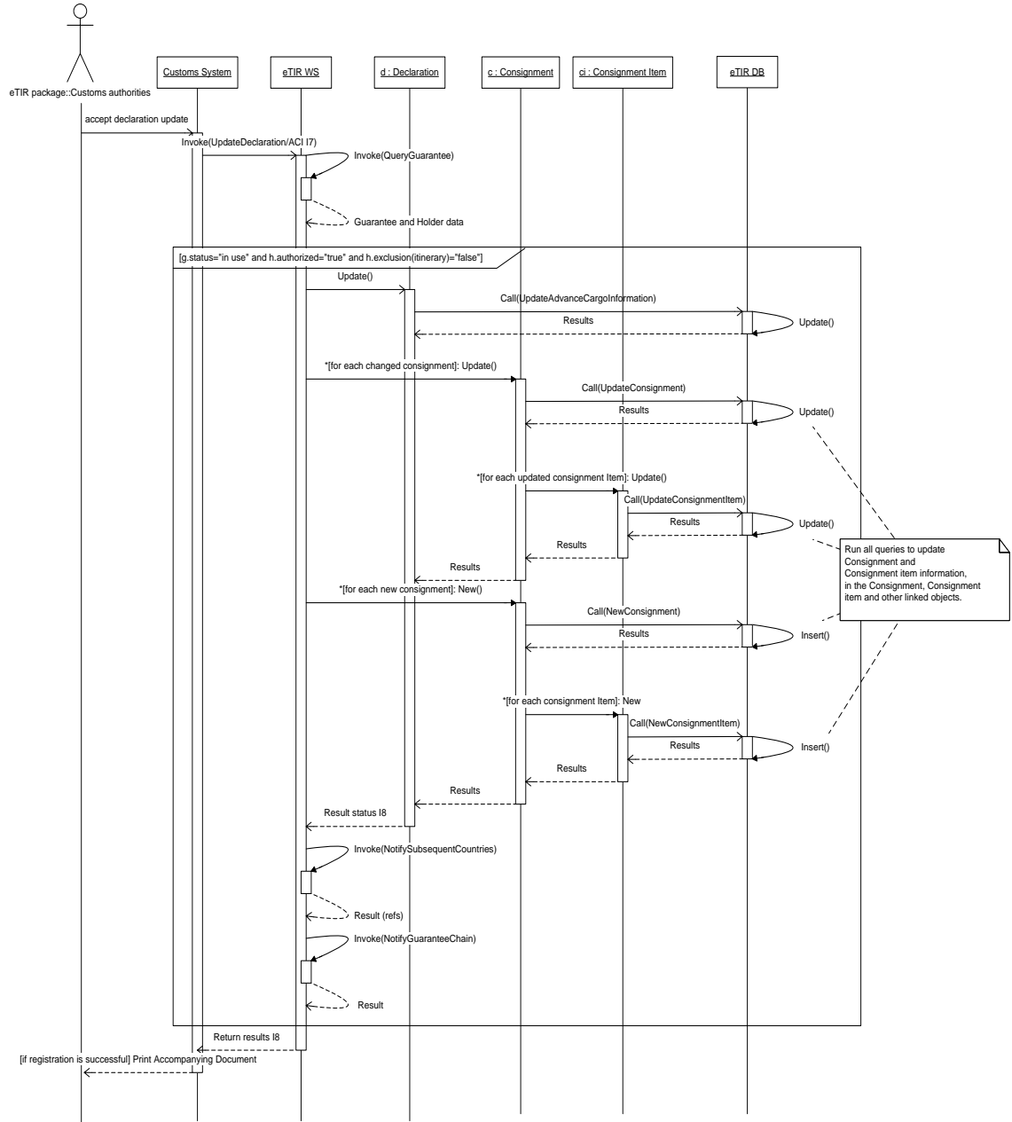
Рис. 3.9 Диаграмма последовательности обновления информации о партии груза (только на английском языке)
