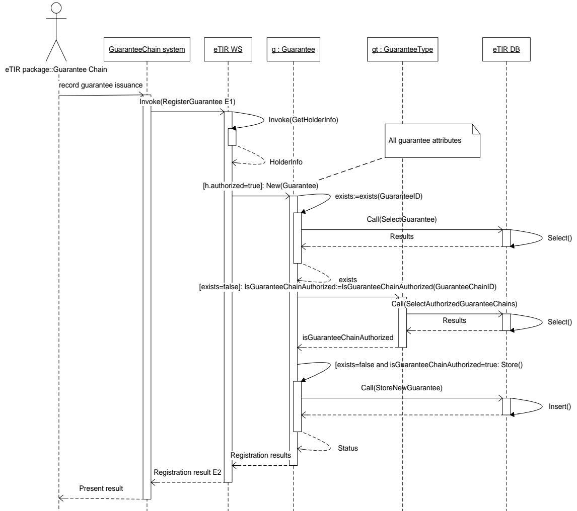
Рис. 3.2 Диаграмма последовательности регистрации гарантии (только на английском языке)
