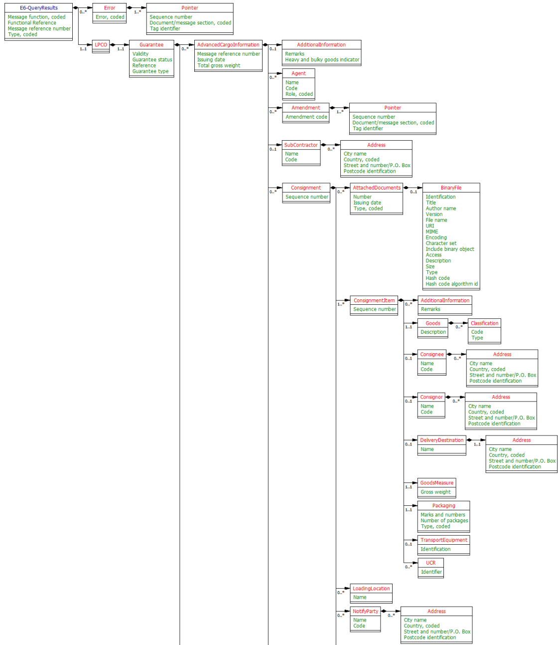
Рис. 3.24: (только на английском языке) Query results UML diagram
