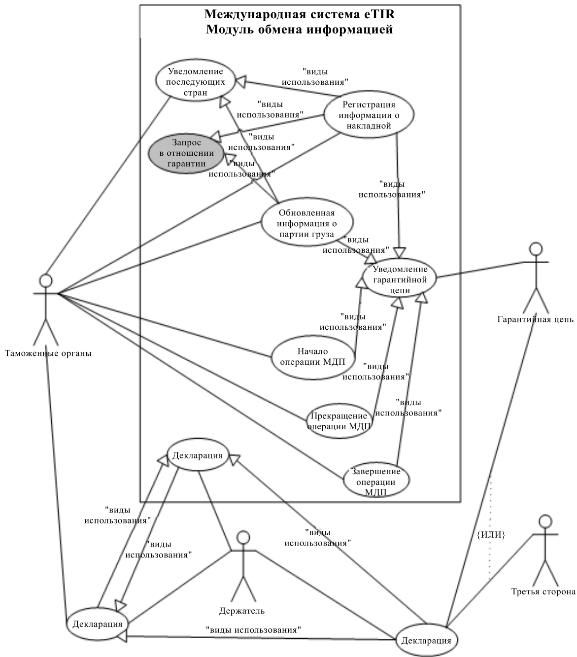
Диаграмма варианта использования обмена данными 1
