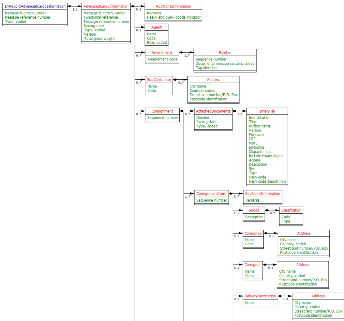
Рис. 3.35: (только на английском языке) Record advanced cargo information UML diagram
