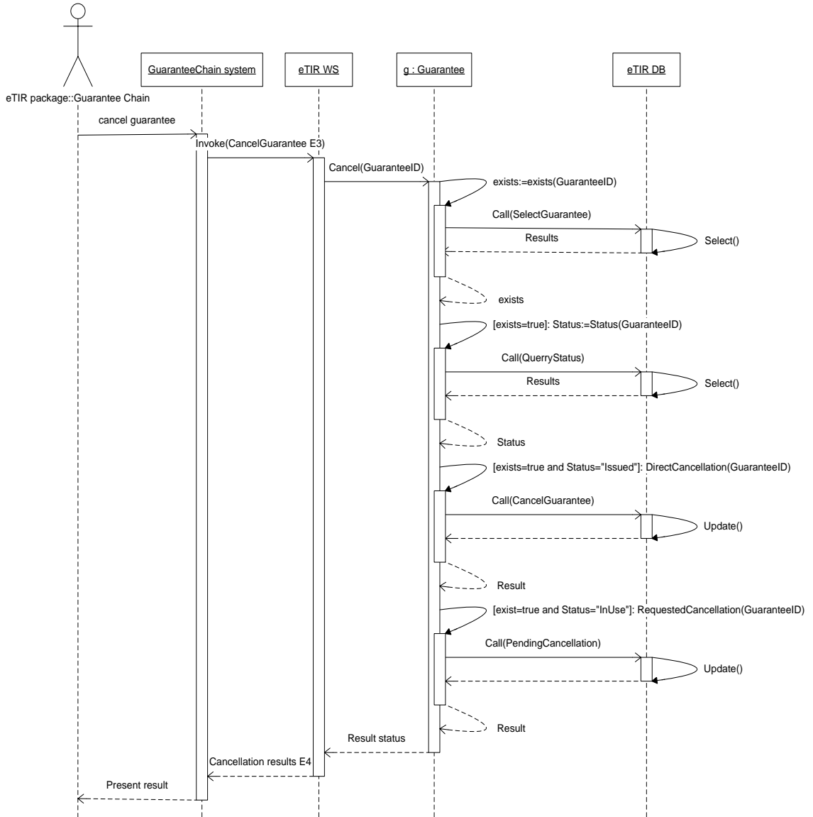
Рис. 3.3 Диаграмма последовательности отмены гарантии (только на английском языке)
