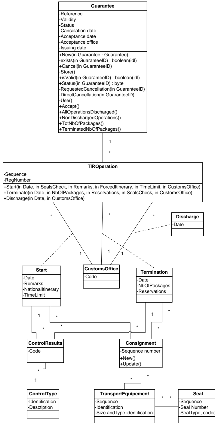
Рис. 3.18 (только на английском языке) Диаграмма класса обмена данными
