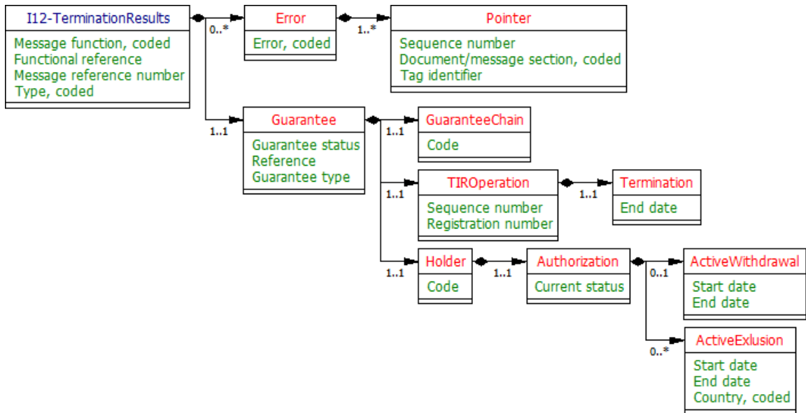
Рис. 3.40: (только на английском языке)
