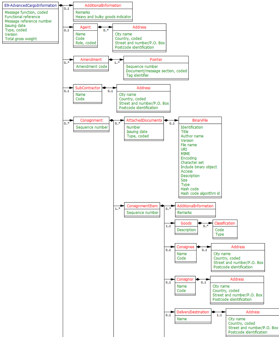
Рис. 3.27: (только на английском языке) Advanced cargo information UML diagram
