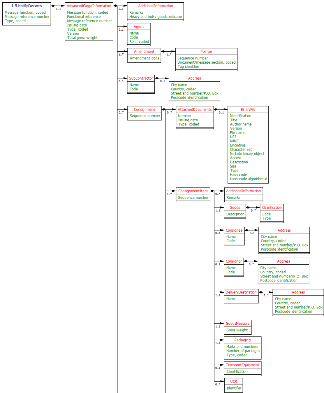
Рис. 3.43: (только на английском языке) Notify Customs UML diagram
