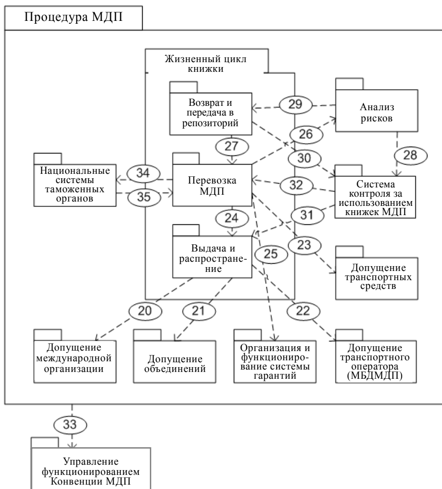
Рис. 1.2 Пакетная диаграмма процедуры МДП
