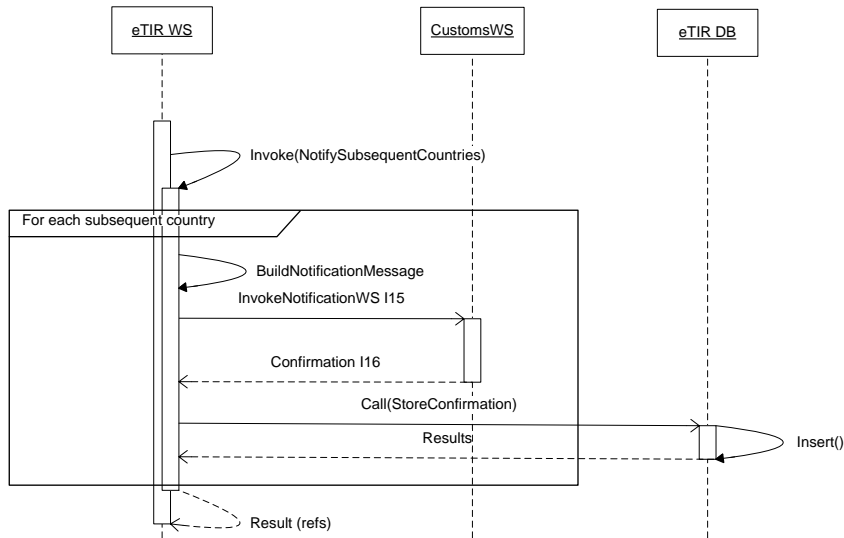
Рис. 3.14 Диаграмма последовательности уведомления последующих стран (только на английском языке)
