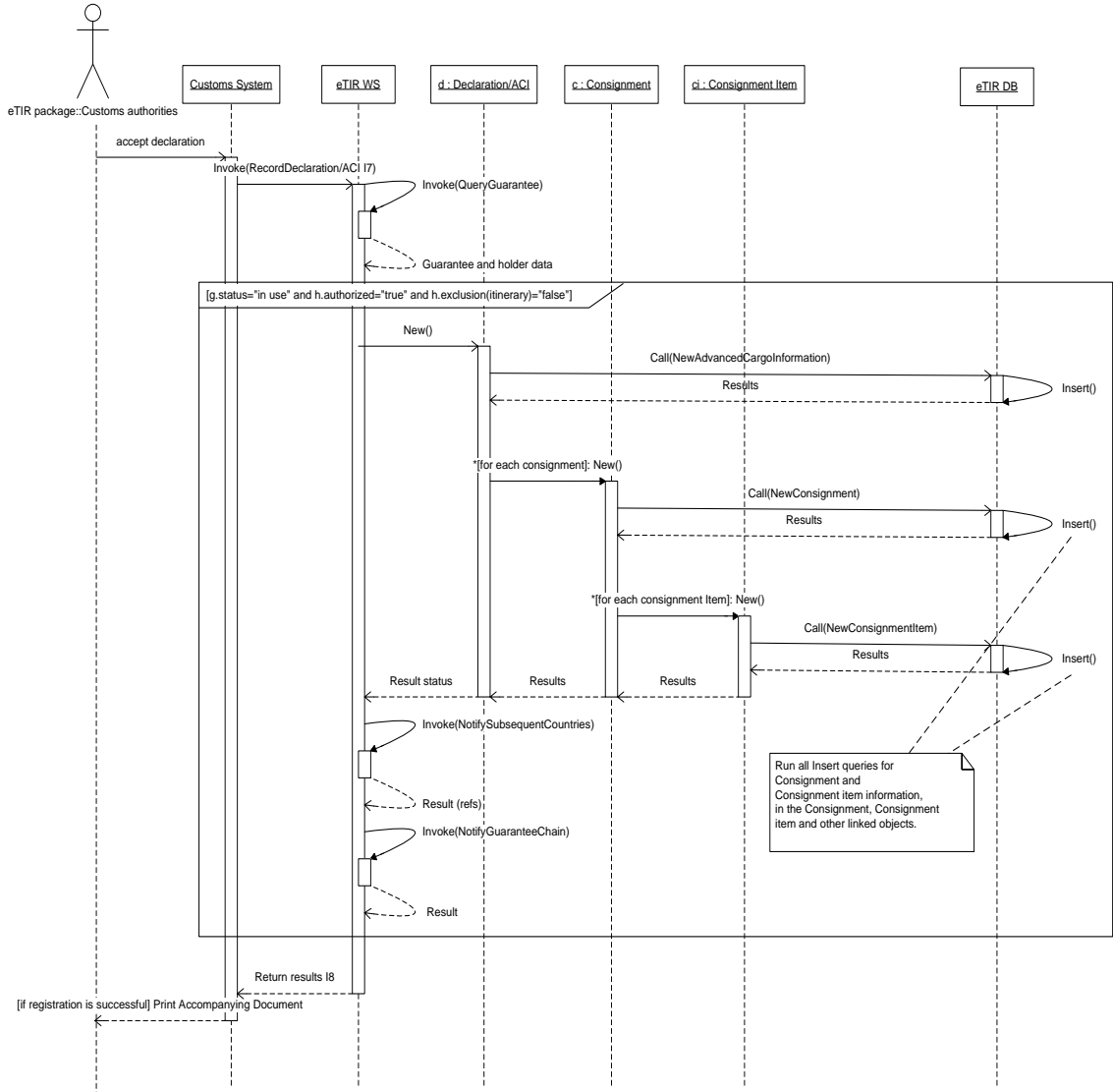
Рис. 3.8 Диаграмма последовательности регистрации информации о партии груза (только на английском языке)
