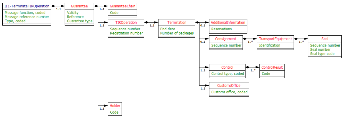
Рис. 3.39: (только на английском языке) Terminate TIR operation UML diagram
