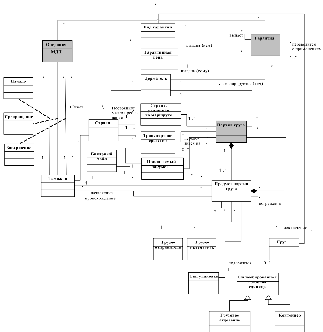
Рис. 2.19 Общая диаграмма классов eTIR
