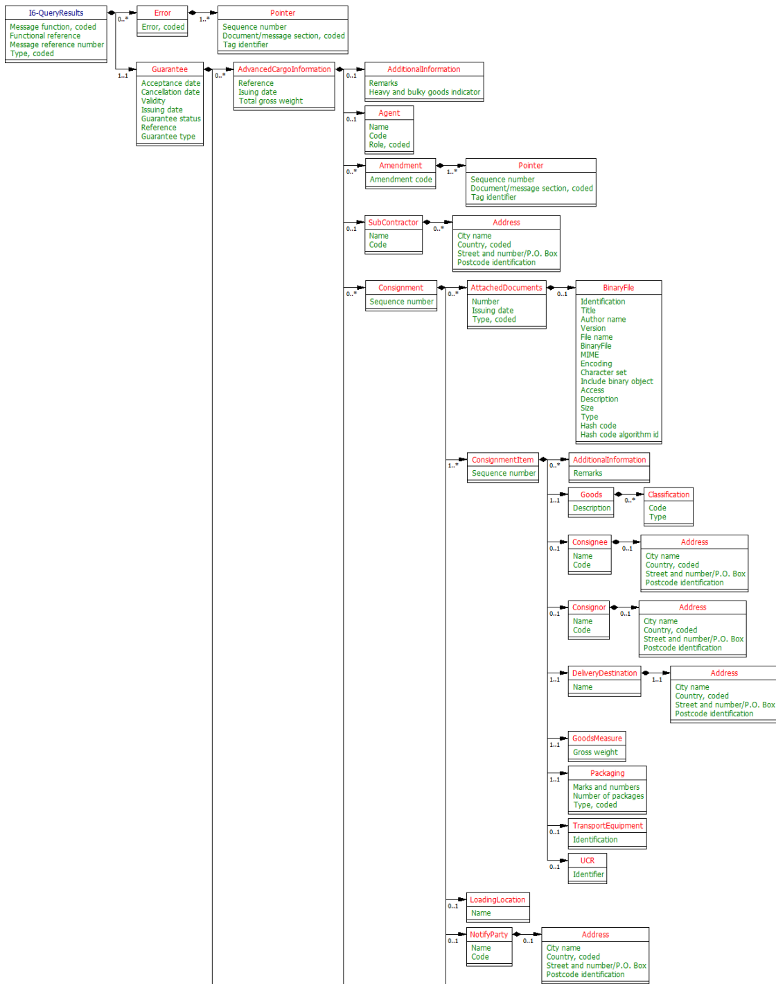
Рис. 3.34: (только на английском языке) Query results UML diagram
