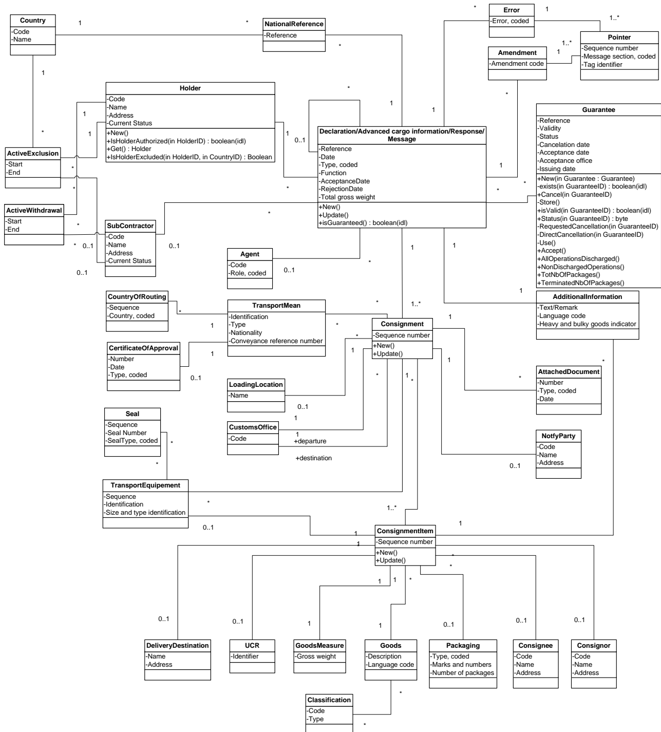
Рис. 3.17 (только на английском языке) Диаграмма класса декларации
