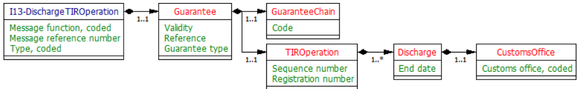
Рис. 3.41: (только на английском языке) Discharge TIR operation UML diagram
