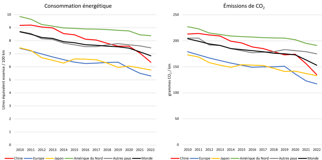
Figure II Tendances de la consommation énergétique des voitures particulières et utilitaires légers
