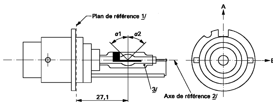
Figure 4 – Catégorie D4S – Type à broche – Culot P32d-5
