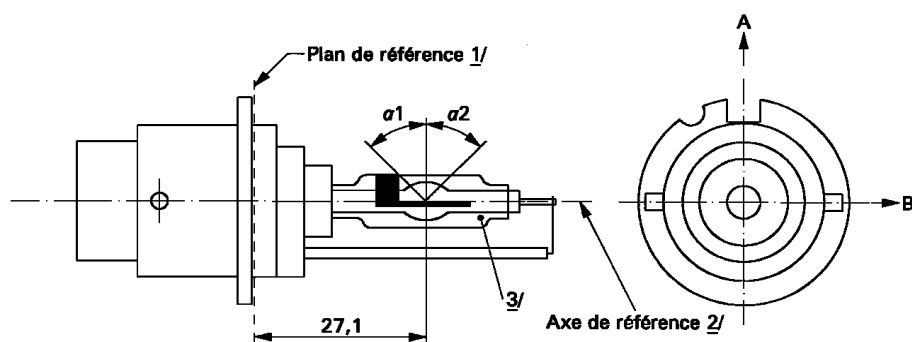
Figure 2 – Catégorie D2S – Type à broche – Culot P32d-2
