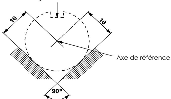
Figure 5 – Définition de l'axe de référence 1/
