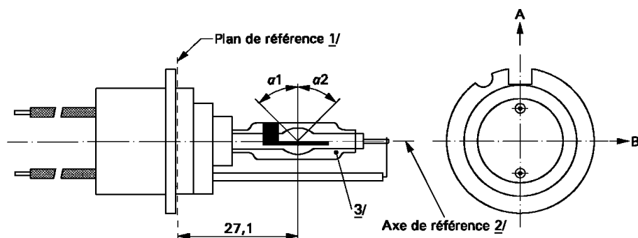
Figure 1 – Catégorie D1S – Type à fils – Culot PK32d-2
