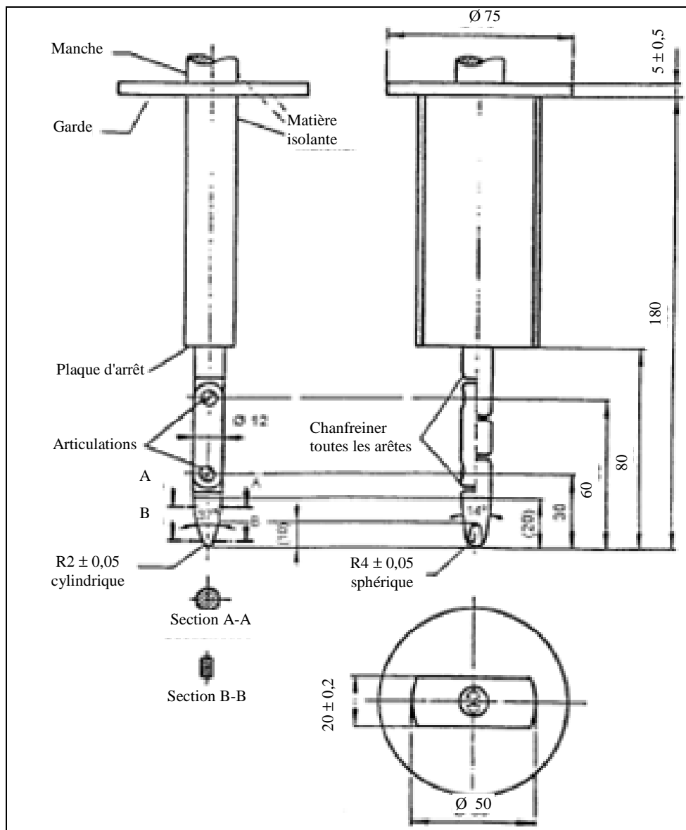
Figure 1 Doigt d'épreuve articulé
