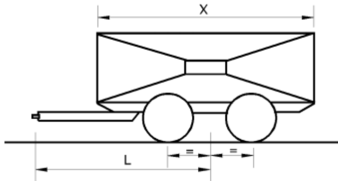
Figure 27 Dimensions de la remorque à essieu(x) médian(s)
