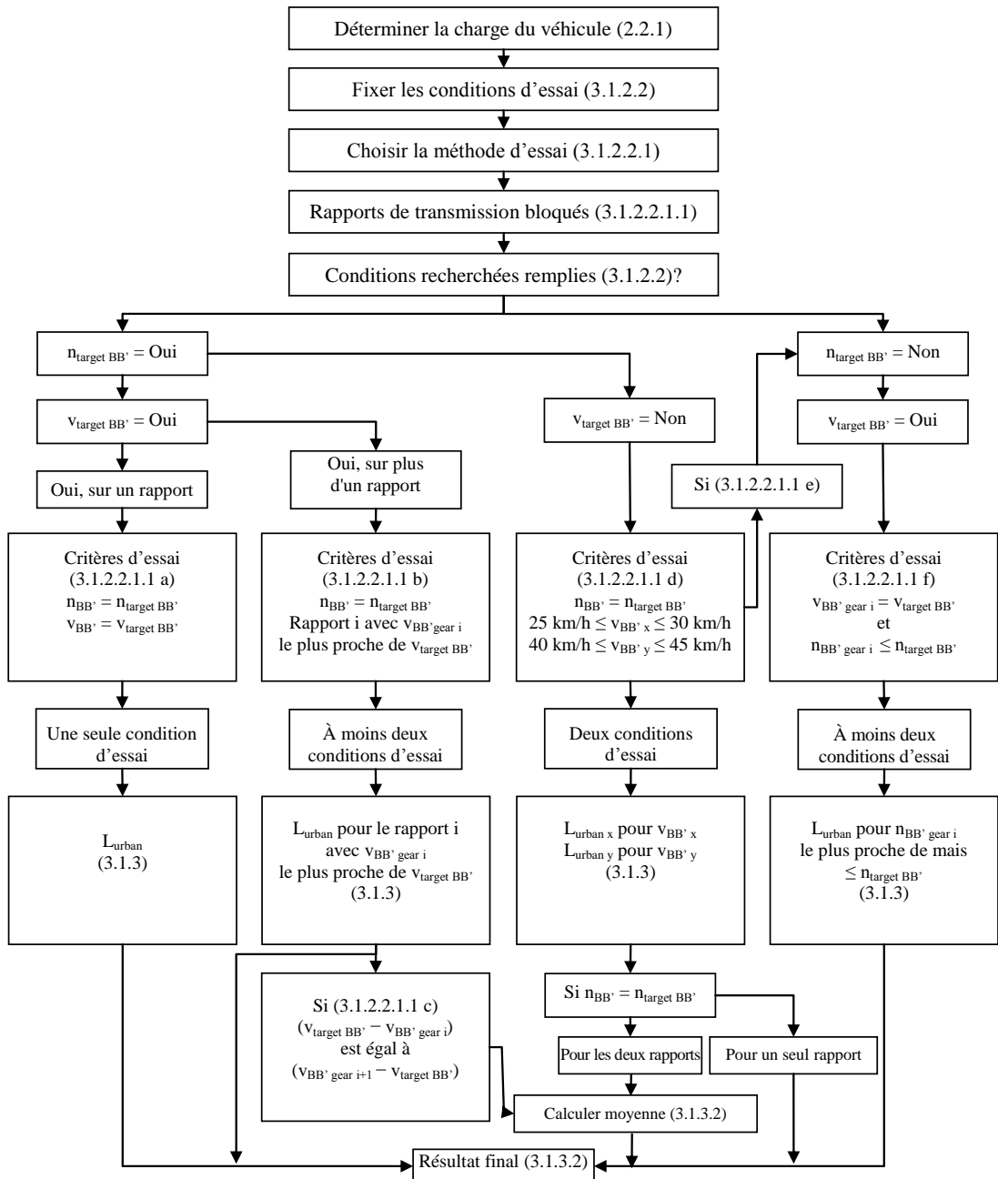
Figure 4a* Diagramme de décision pour les véhicules soumis à essai conformément aux dispositions du paragraphe 3.1.2.2 de l'annexe 3 du présent Règlement – Essai rapports bloqués
