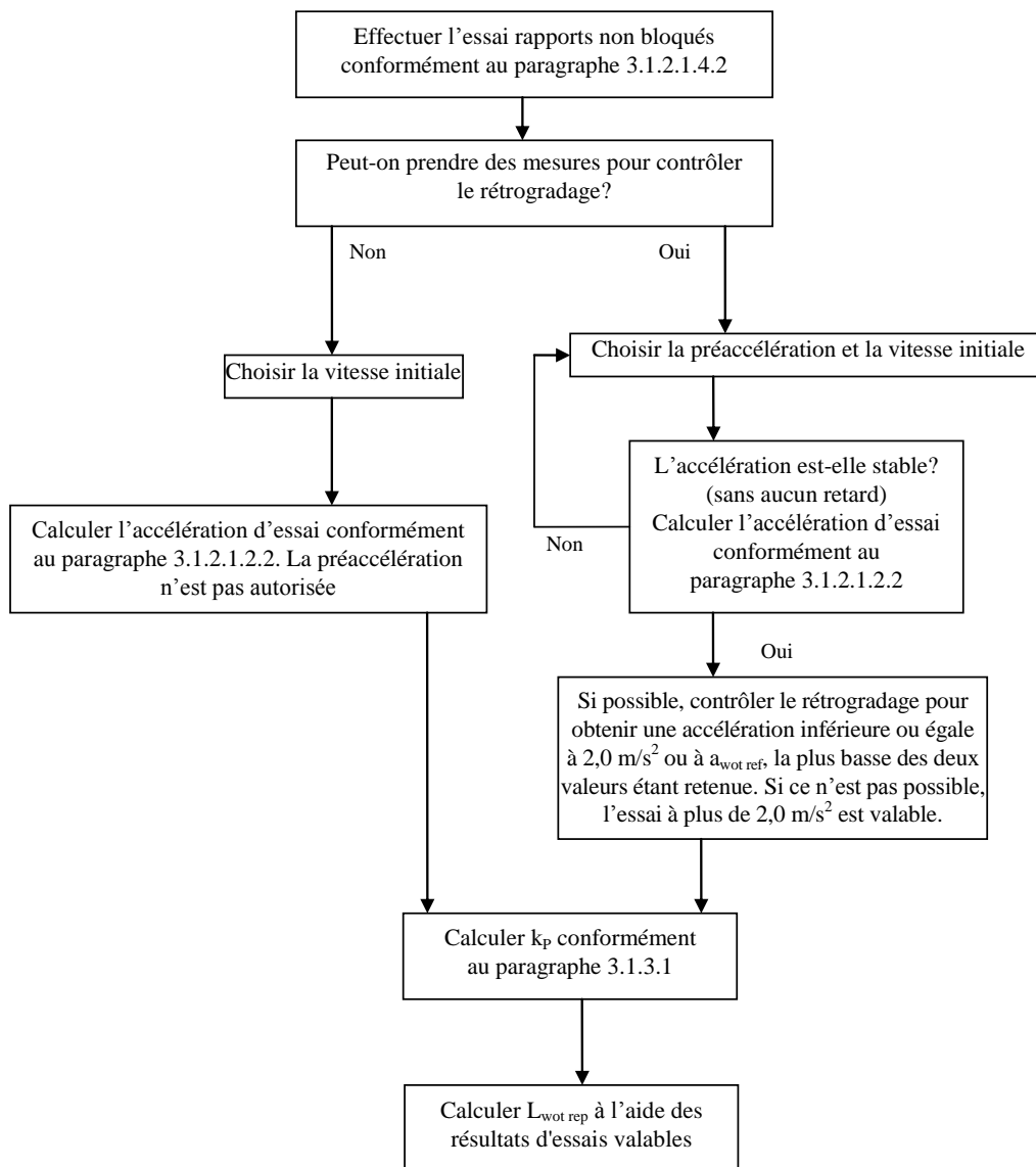
Figure 3e Diagramme de décision pour les véhicules soumis à essai conformément aux dispositions du paragraphe 3.1.2.1 de l'annexe 3 du présent Règlement – Sélection des rapports avec rapports non bloqués
