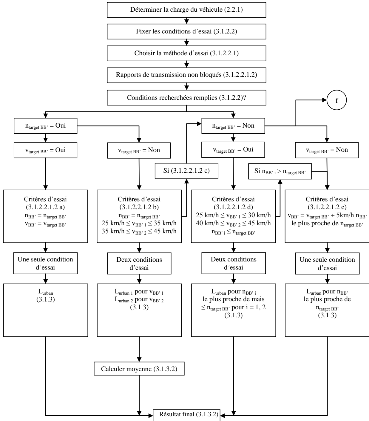
Figure 4b* Diagramme de décision pour les véhicules soumis à essai conformément aux dispositions du paragraphe 3.1.2.2 de l'annexe 3 du présent Règlement – Essai rapports non bloqués – 1 re PARTIE
