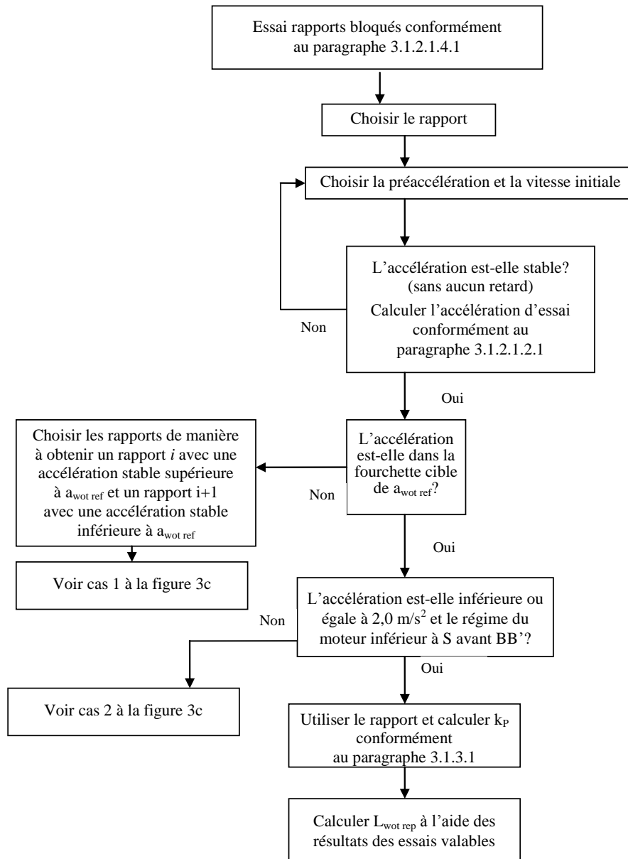
Figure 3b Diagramme de décision pour les véhicules soumis à essai conformément aux dispositions du paragraphe 3.1.2.1 de l'annexe 3 du présent Règlement – Sélection des rapports avec rapports bloqués – 1 re PARTIE
