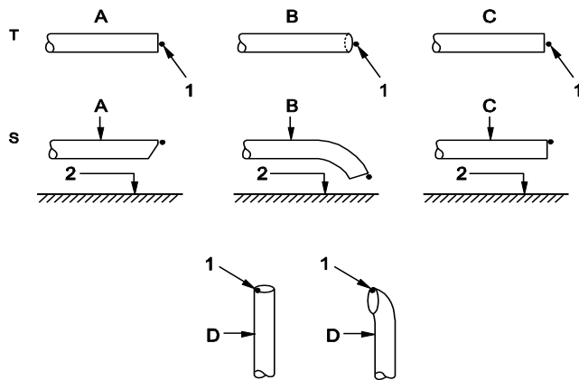
Figure 2 Point de référence pour la mesure du bruit émis par le véhicule à l'arrêt
