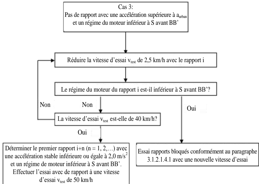
Figure 3d Diagramme de décision pour les véhicules soumis à essai conformément aux dispositions du paragraphe 3.1.2.1 de l'annexe 3 du présent Règlement – Sélection des rapports avec rapports bloqués – 3 e PARTIE
