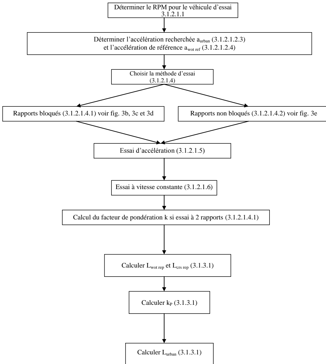
Figure 3a Diagramme d'ordonnancement pour les véhicules soumis à essai conformément aux dispositions du paragraphe 3.1.2.1 de l'annexe 3 du présent Règlement – calcul de L_{urban}
