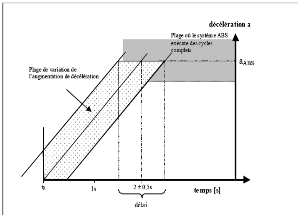
Plage de décélération pour la détermination de F_{ABS} et a_{ABS}
