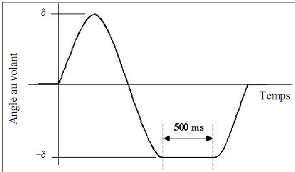
Figure 2 Impulsion Sinus avec palier
