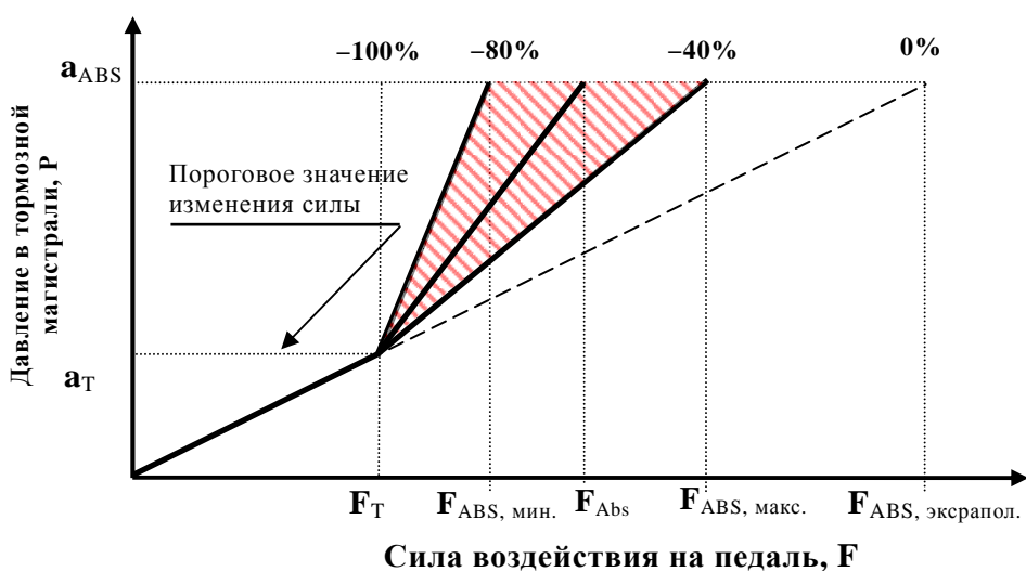
Рис. 1b Характеристика изменения силы воздействия на педаль, необходимой для достижения максимального замедления в случае СВТ категории "А"
