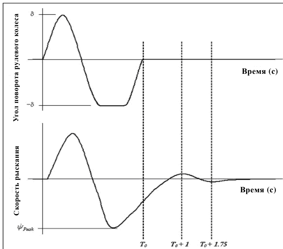
Рис. 1 Данные, определяющие положение рулевого колеса и скорость рыскания, которые используют для оценки боковой устойчивости
