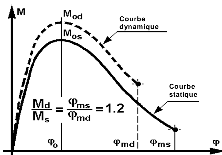
Figure A8.A1.2 – Courbe dynamique déduite de la courbe statique pour une articulation plastique
