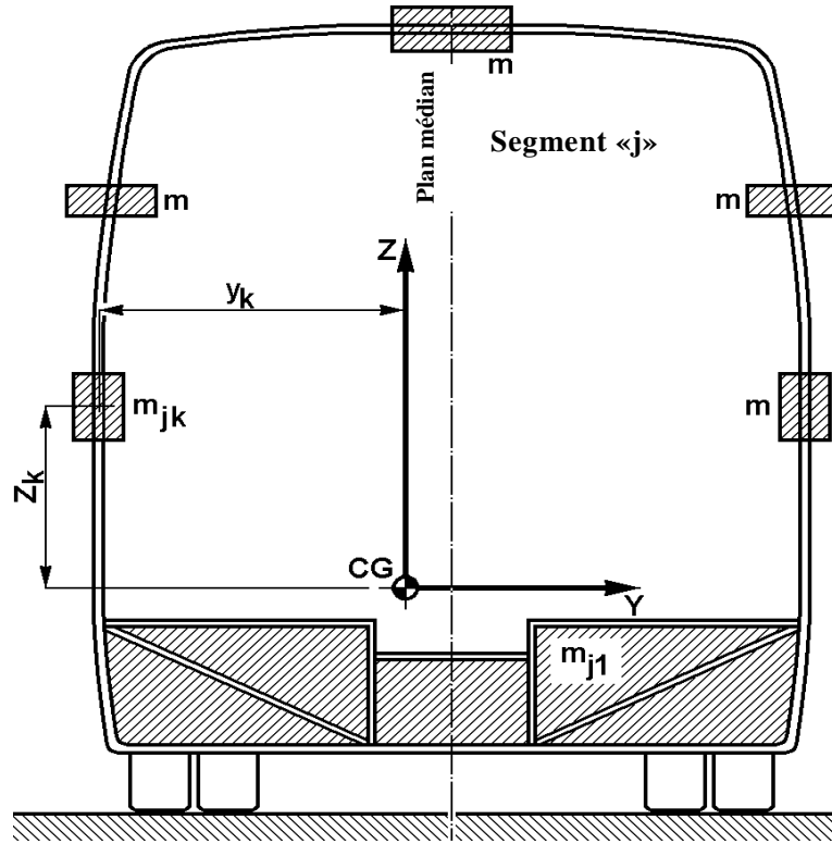
Figure A4.4 – Répartition des masses dans la section transversale d'un segment
