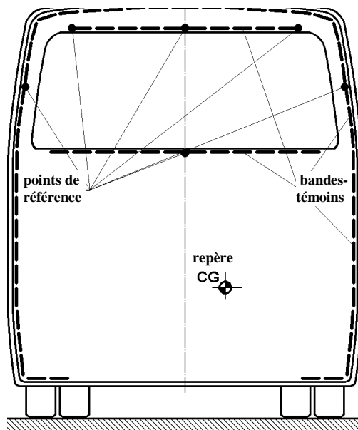
Figure A5.3b – Marquage recommandé pour la position du centre de gravité et le contour du véhicule
