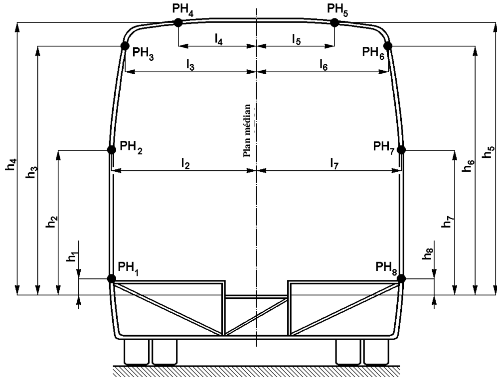
Figure A8.1 – Paramètres géométriques des articulations plastiques d'un segment
