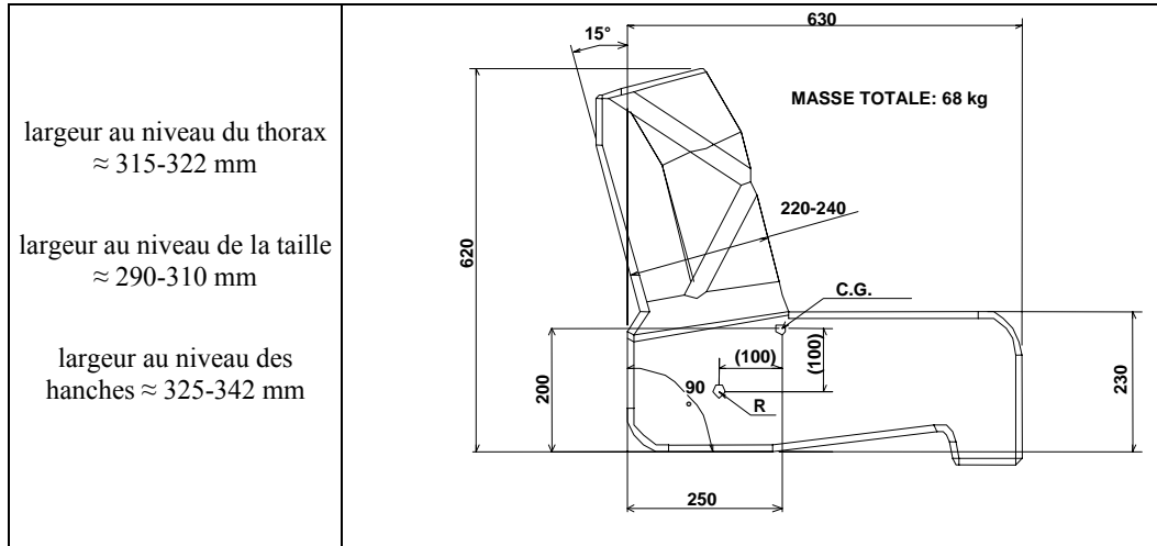
Figure A5.2 – Dimensions du mannequin anthropomorphe
