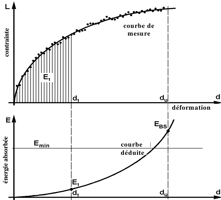
Figure A7.2 – Énergie absorbée par la section de caisse, déduite de la courbe de mesure contrainte/déformation
