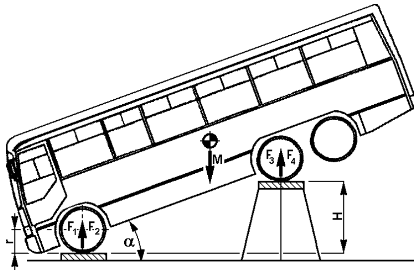
Figure A3.3 – Détermination de la hauteur du centre de gravité
