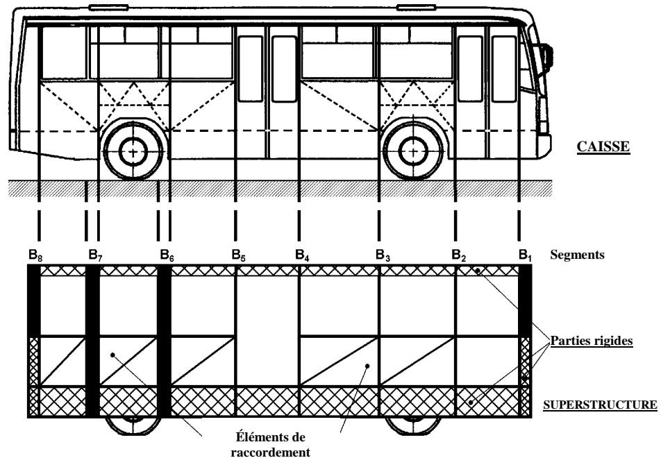
Figure A4.1 – Définition de la superstructure à partir de la caisse
