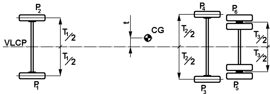
Figure A3.2 – Position transversale du centre de gravité
