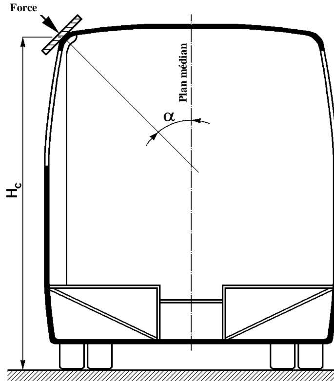
Figure A8.2 – Application de la force à la superstructure
