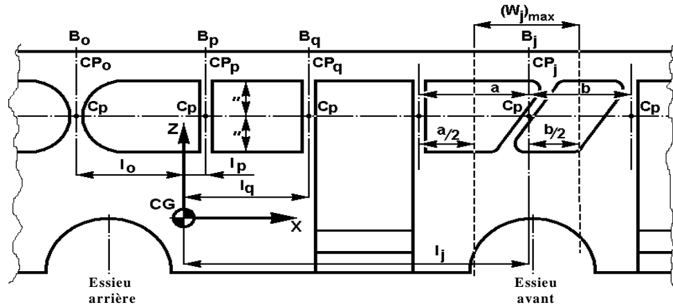
Figure A4.2 – Définition de la longueur d'un segment
