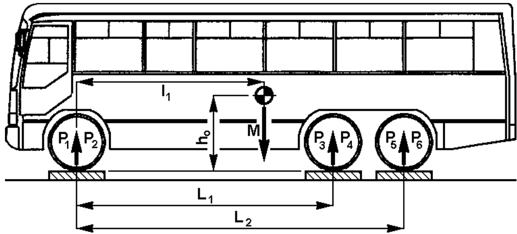
Figure A3.1 – Position longitudinale du centre de gravité
