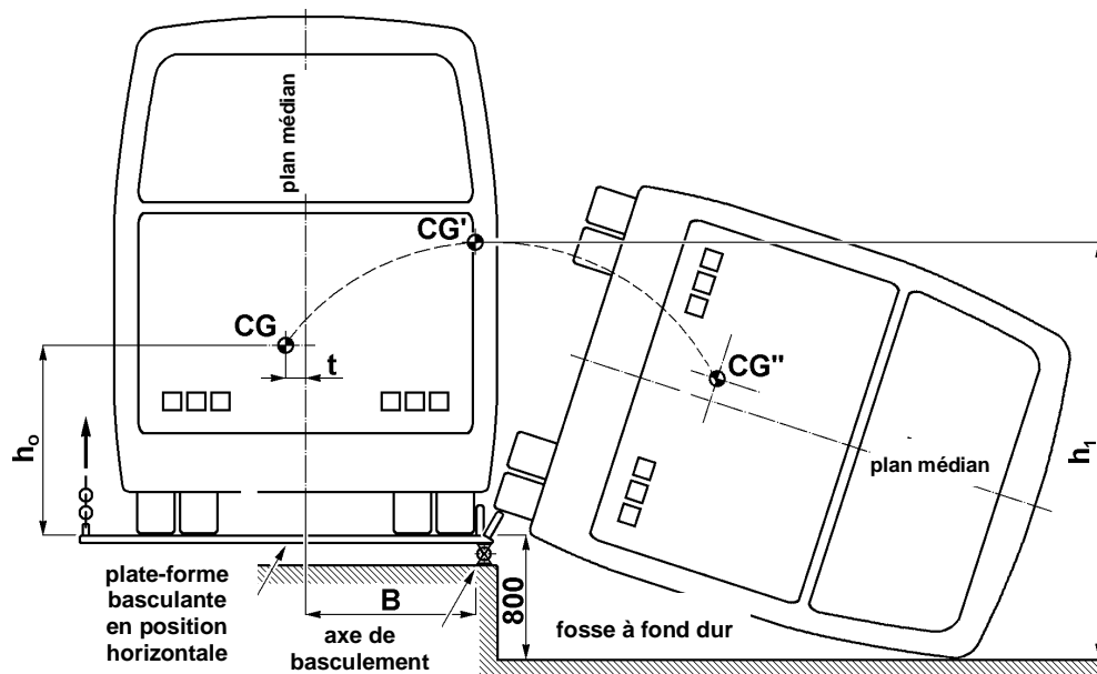
Figure 3 – Représentation de l'essai de renversement sur un véhicule complet, indiquant la trajectoire du centre de gravité depuis la position horizontale jusqu'à la position finale en passant par la position d'équilibre instable
