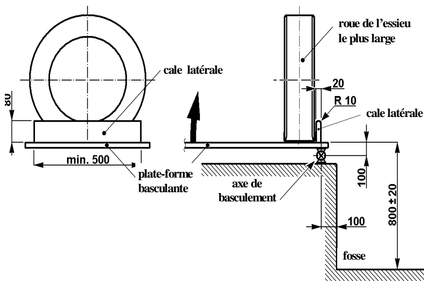
Figure A5.1 – Cotes géométriques du banc de basculement
