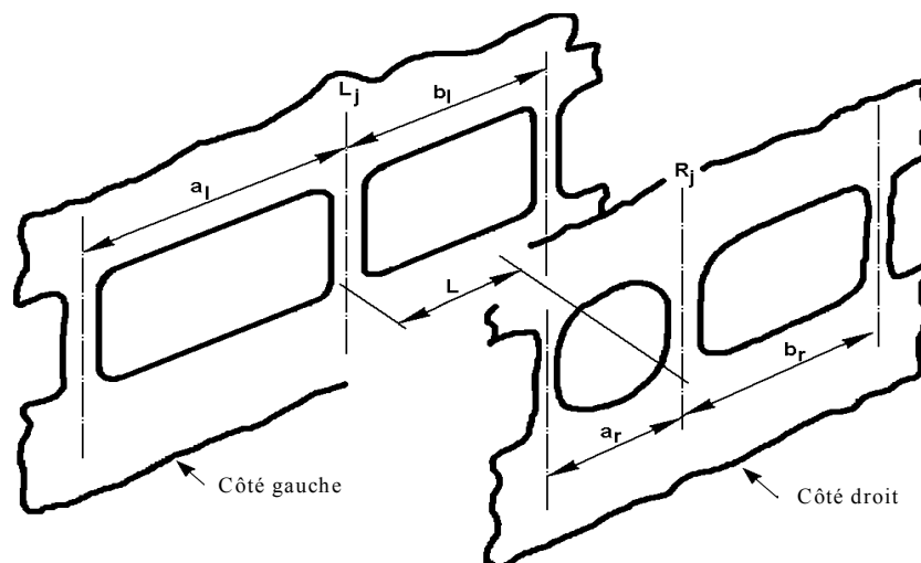
Figure A4.3 – Définition de la longueur d'un segment lorsque les montants de chaque côté du segment ne sont pas dans un même plan transversal
