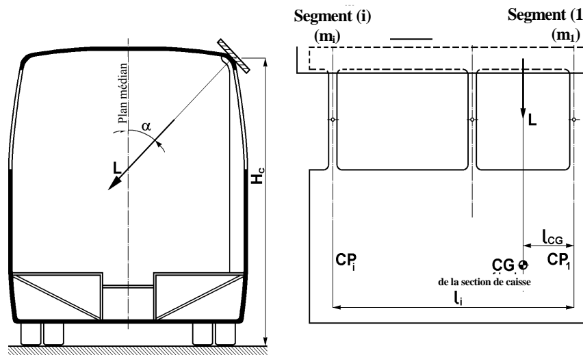
Figure A7.1 – Application de la force à la section de caisse
