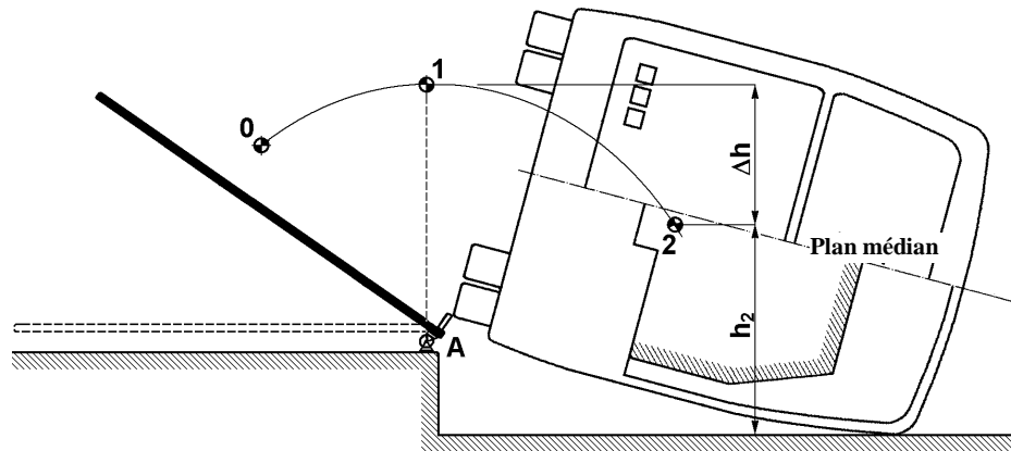
Figure A7.A1.2 – Détermination du mouvement vertical du centre de gravité du véhicule
