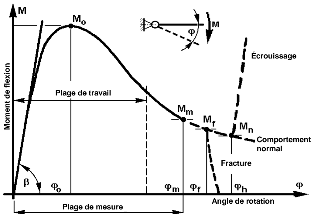
Figure A8.A1.1 – Courbe caractéristique d'une articulation plastique
