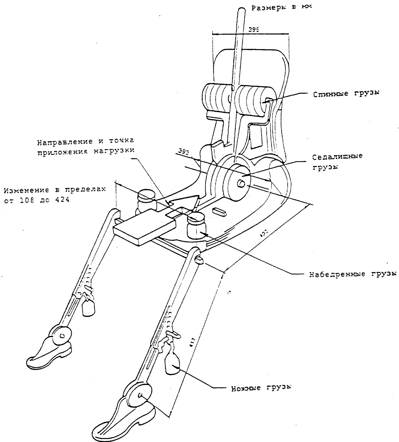
Рисунок 2 - Размеры элементов механизма 3-D и распределения грузов
