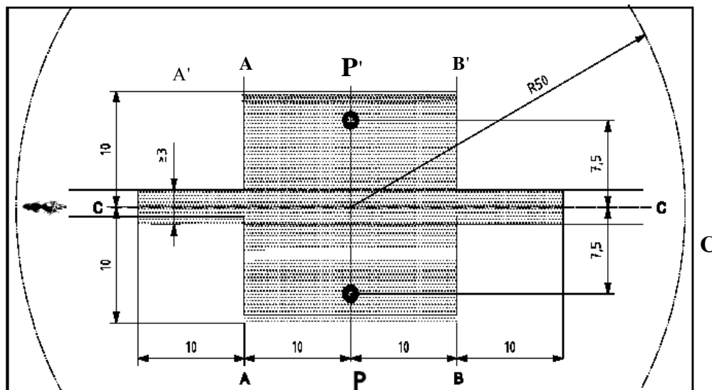
Рис. 1 Минимальные требования в отношении зоны с испытательным покрытием. Заштрихованная часть называется "зоной испытания"
