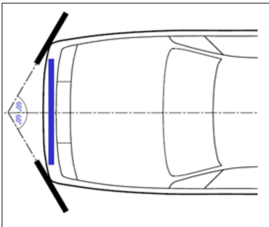
Figure 5D Détermination de la zone d'impact du pare-chocs (noter que les gabarits de coin doivent être déplacés verticalement et horizontalement de sorte qu'ils entrent en contact avec le contour extérieur ou le tablier avant du véhicule)
