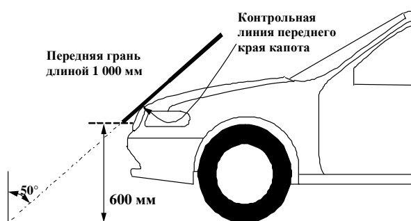
Рис. 1 Контрольная линия переднего края капота
