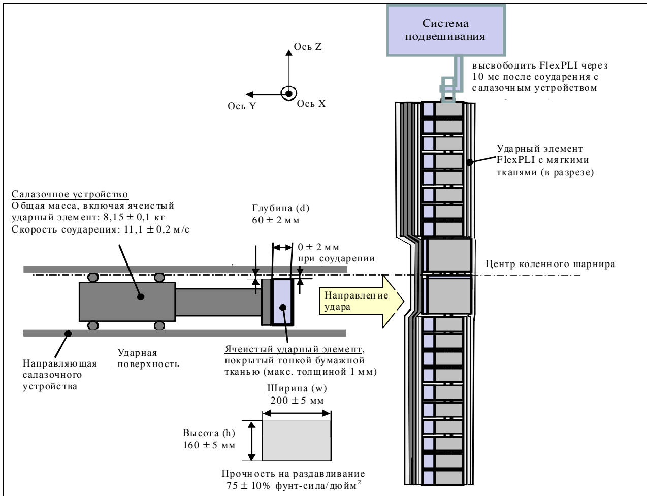
Рис. 7 Ударный элемент в виде гибкой модели нижней части ноги: испытательная установка для проведения динамического испытания ударного элемента в виде модели нижней части ноги в целях сертификации (обратное испытание, см. пункт 1.4.3.1 настоящего приложения)
