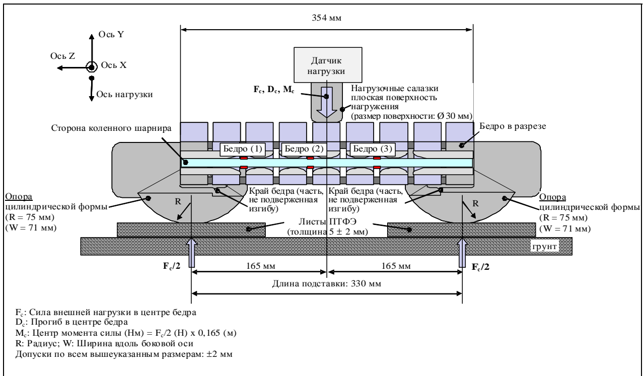
Рис. 3 Ударный элемент в виде гибкой модели нижней части ноги: испытательная установка для проведения испытания бедра при статических сертификационных испытаниях (см. пункт 1.2.4 настоящего приложения)
