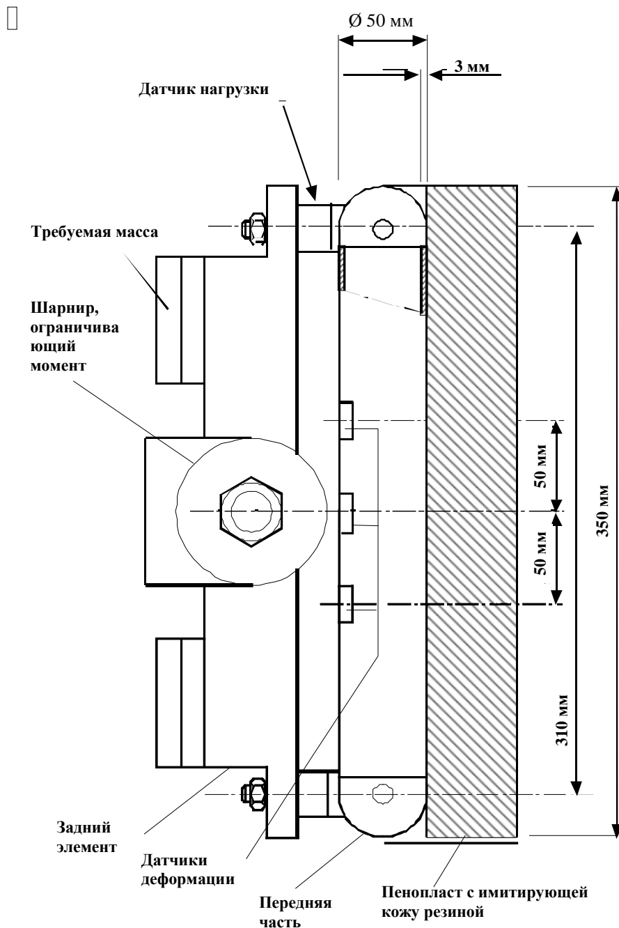
Рис. 4 Ударный элемент в виде модели верхней части ноги
