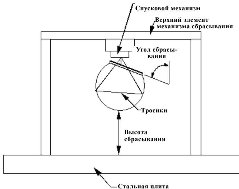
Рис. 9 Испытательная установка для проведения динамического испытания ударного элемента в виде модели головы на соответствие биомеханическим характеристикам
