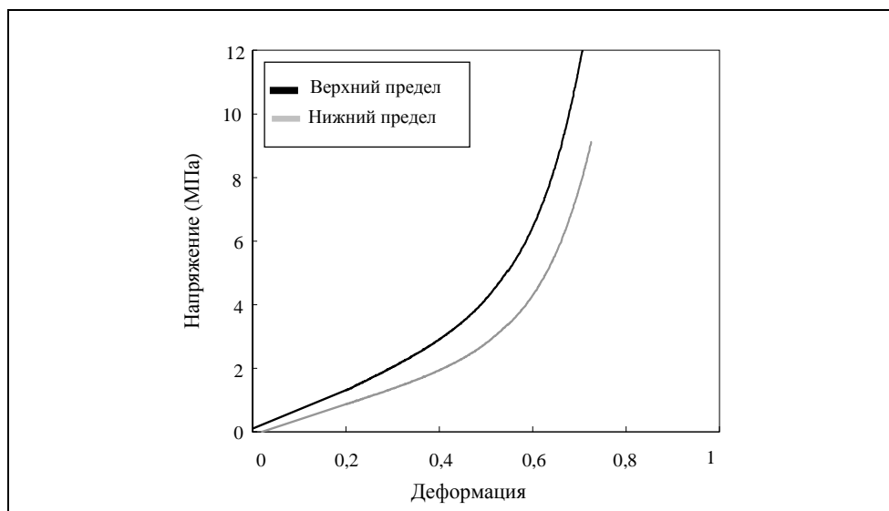
Рис. 2 Ударный элемент в виде гибкой модели ноги: характеристики компрессии элементов, изготовленных с использованием имитирующих мягкие ткани и кожу материалов
