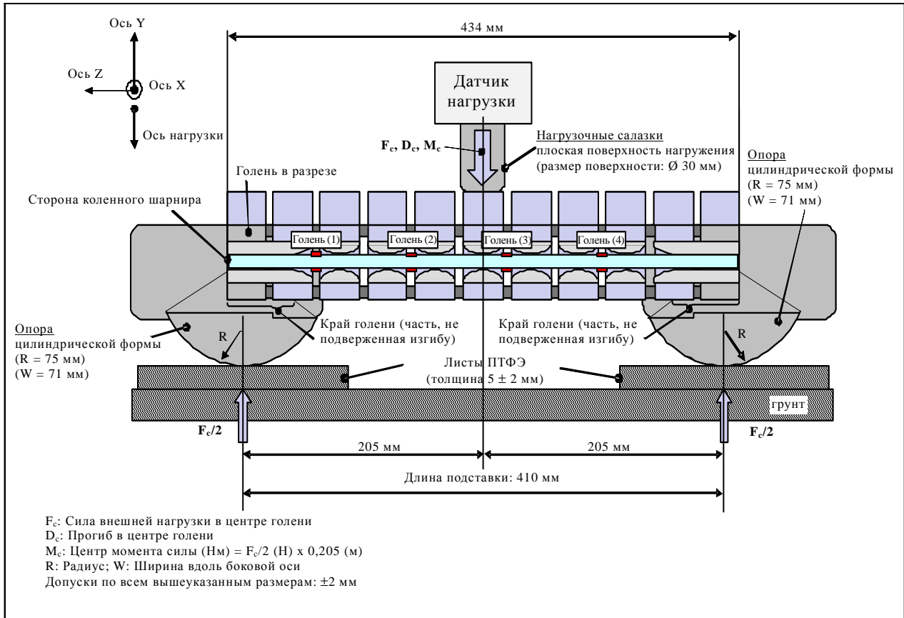
Рис. 4 Ударный элемент в виде гибкой модели нижней части ноги: испытательная установка для проведения испытания голени при статических сертификационных испытаниях (см. пункт 1.2.4 настоящего приложения)
