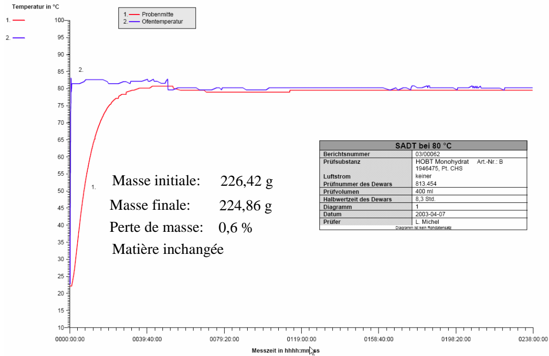
Figure 6: Épreuve de stockage avec accumulation de chaleur (épreuve H.4 de l'ONU) à 80 °C
