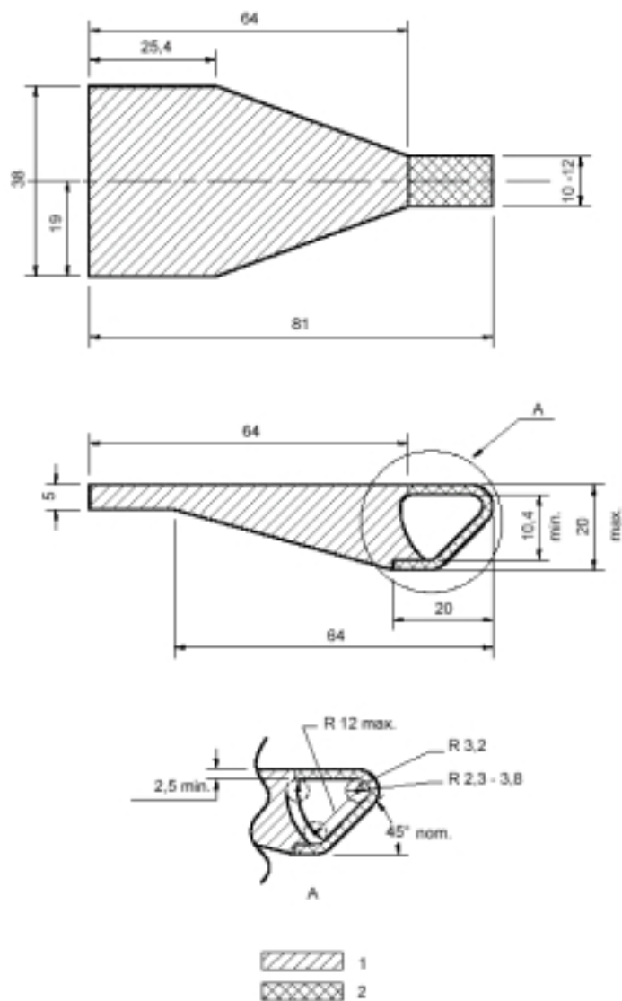
Légende 1 Structure environnante (si présente) 2 Zone dans laquelle le profil de l'interface du crochet de sangle supérieure doit être entièrement situé
