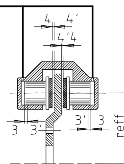
Frein à disque
