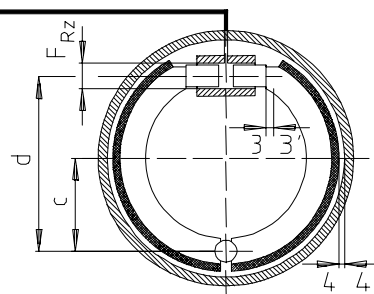
Frein à tambour
