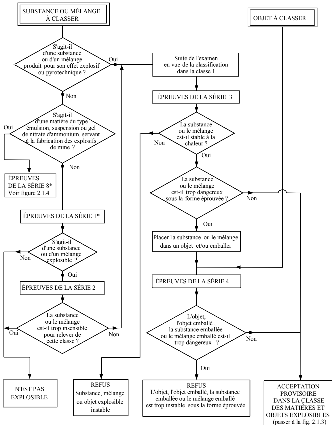
Figure 2.1.2: Procédure d'acceptation temporaire d'une substance, d'un mélange ou d'un objet dans la classe des matières et objets explosibles (Classe 1)
