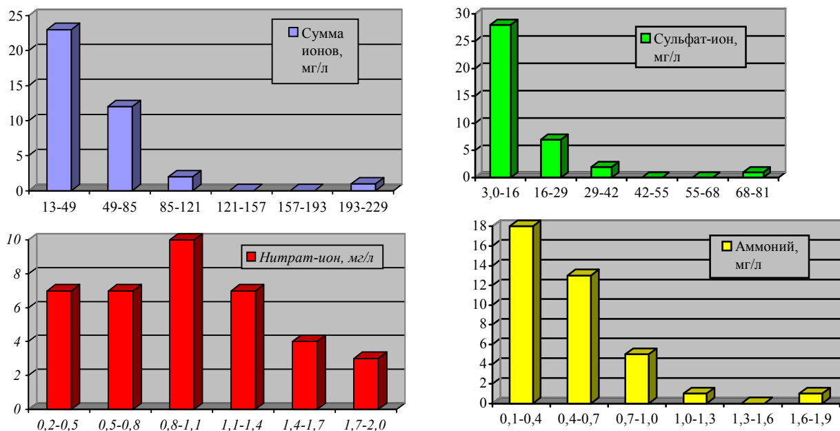
Рисунок II-4: Распределение содержания отдельных показателей атмосферных осадков по метеостанциям по данным 2002 г.
