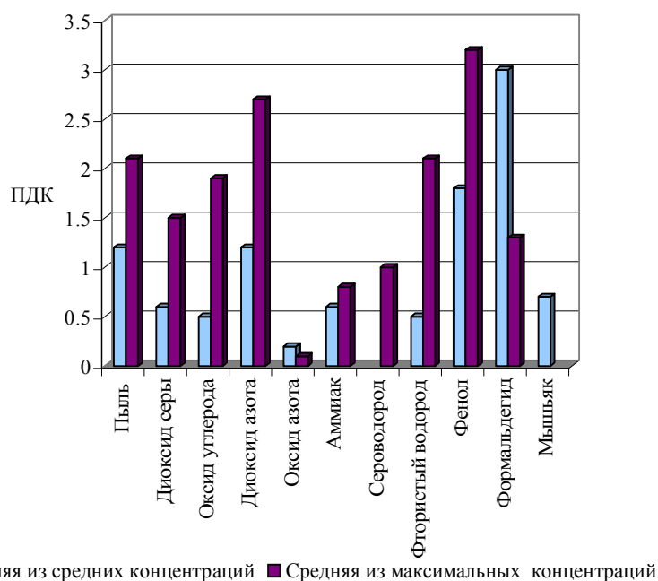
Рисунок II-2: Средние концентрации примесей (кратные ПДК) по городам Республики Казахстан в 2002г.
